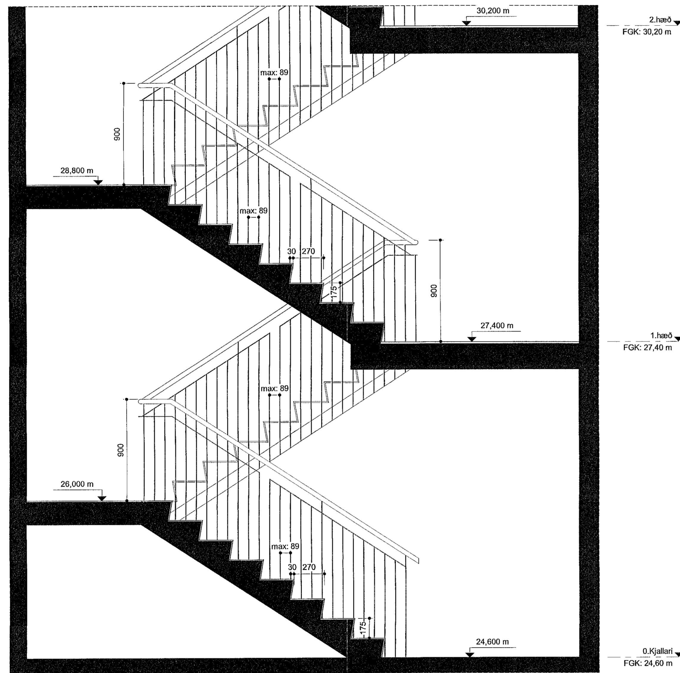
Stigi - Snið 1-1 - 1.hluti
