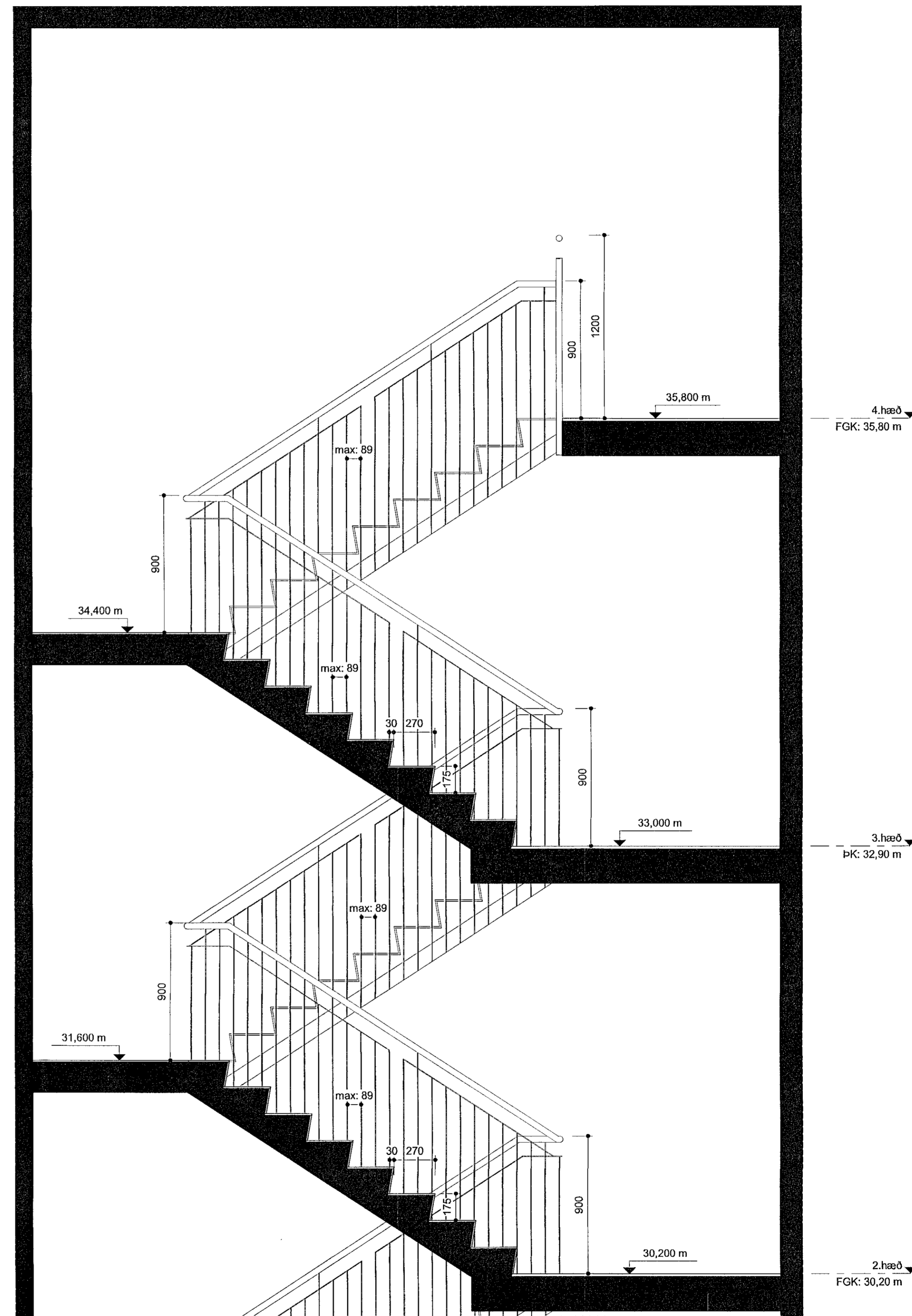
Stigi - Snið 1-1 - 2.hluti
