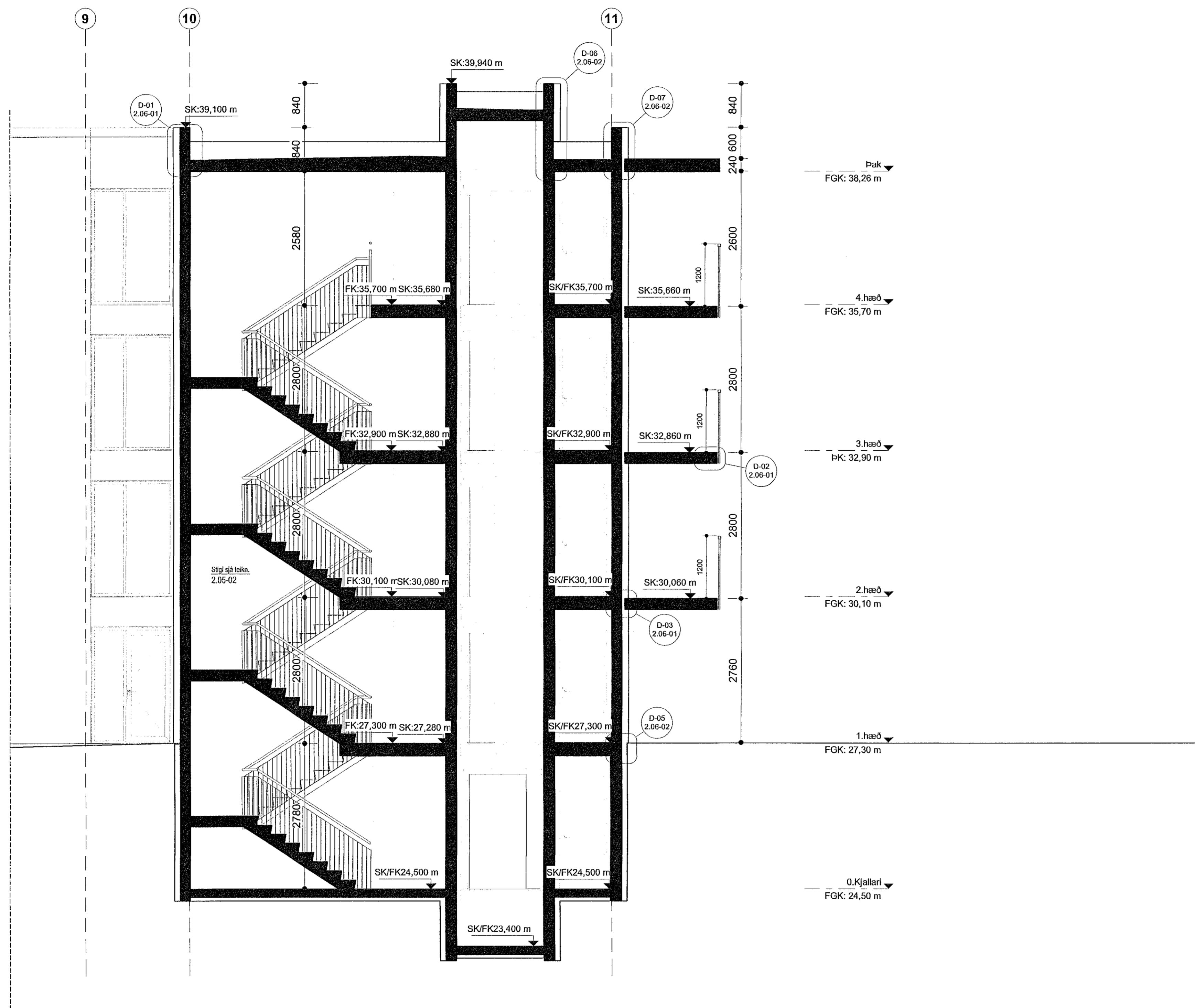
Snið B-B
