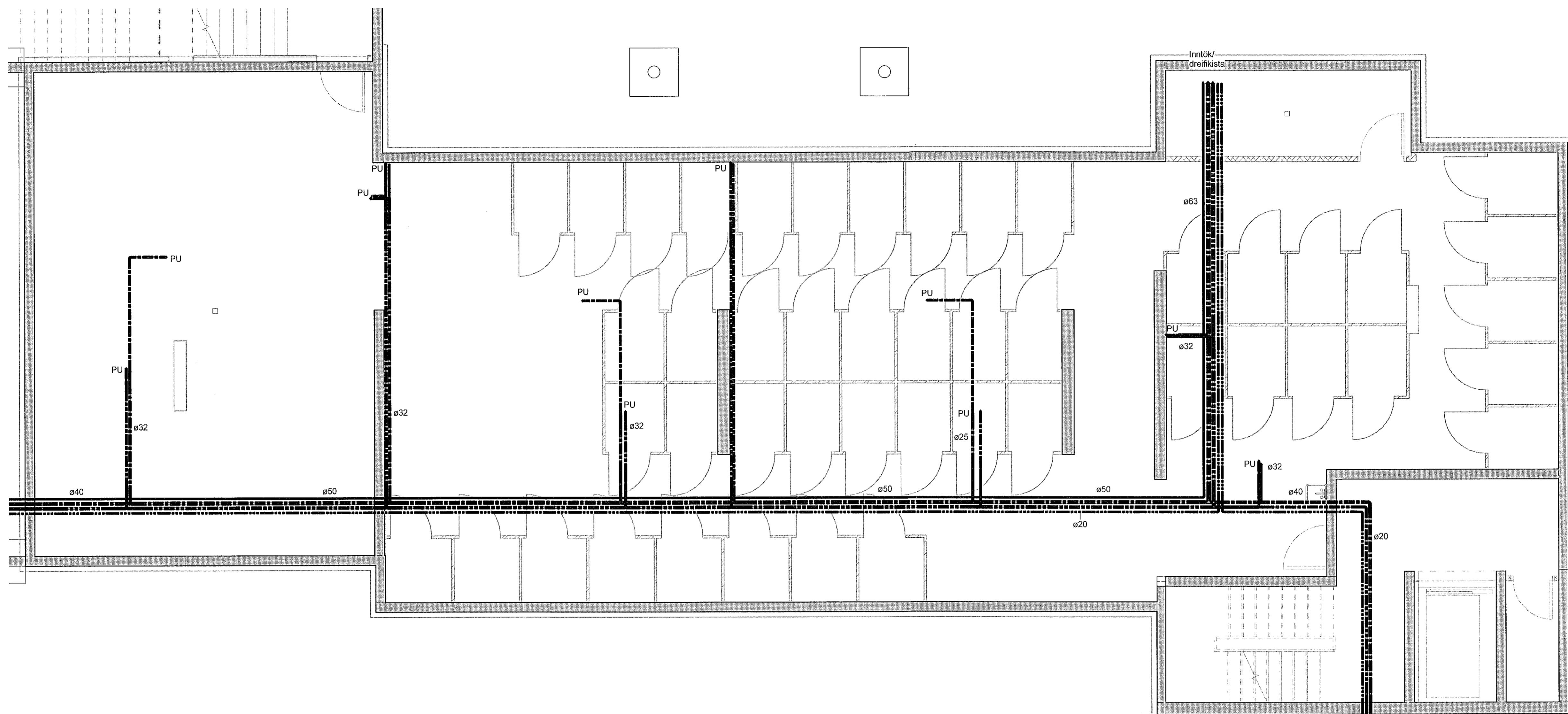
1 Kjallari - 2 1 : 50
