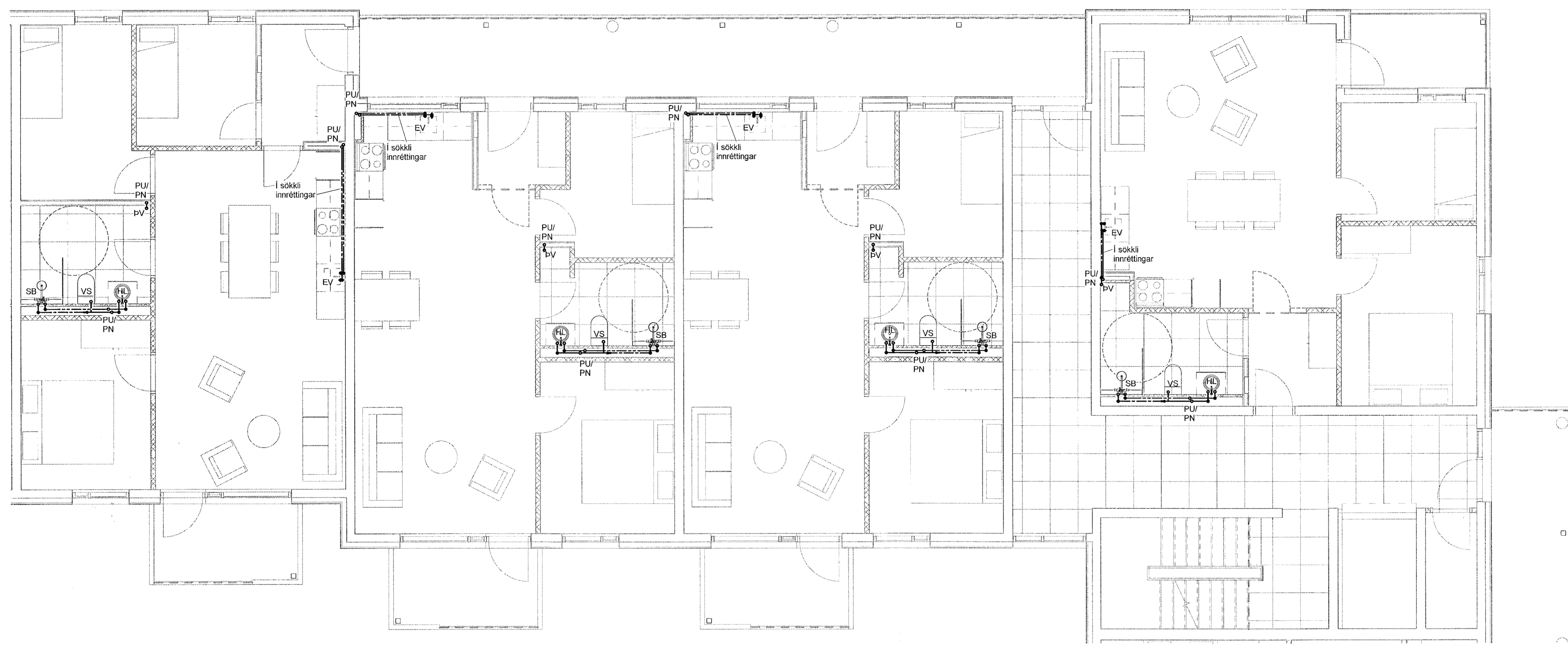
1 2. hæð - 2 1 : 50
