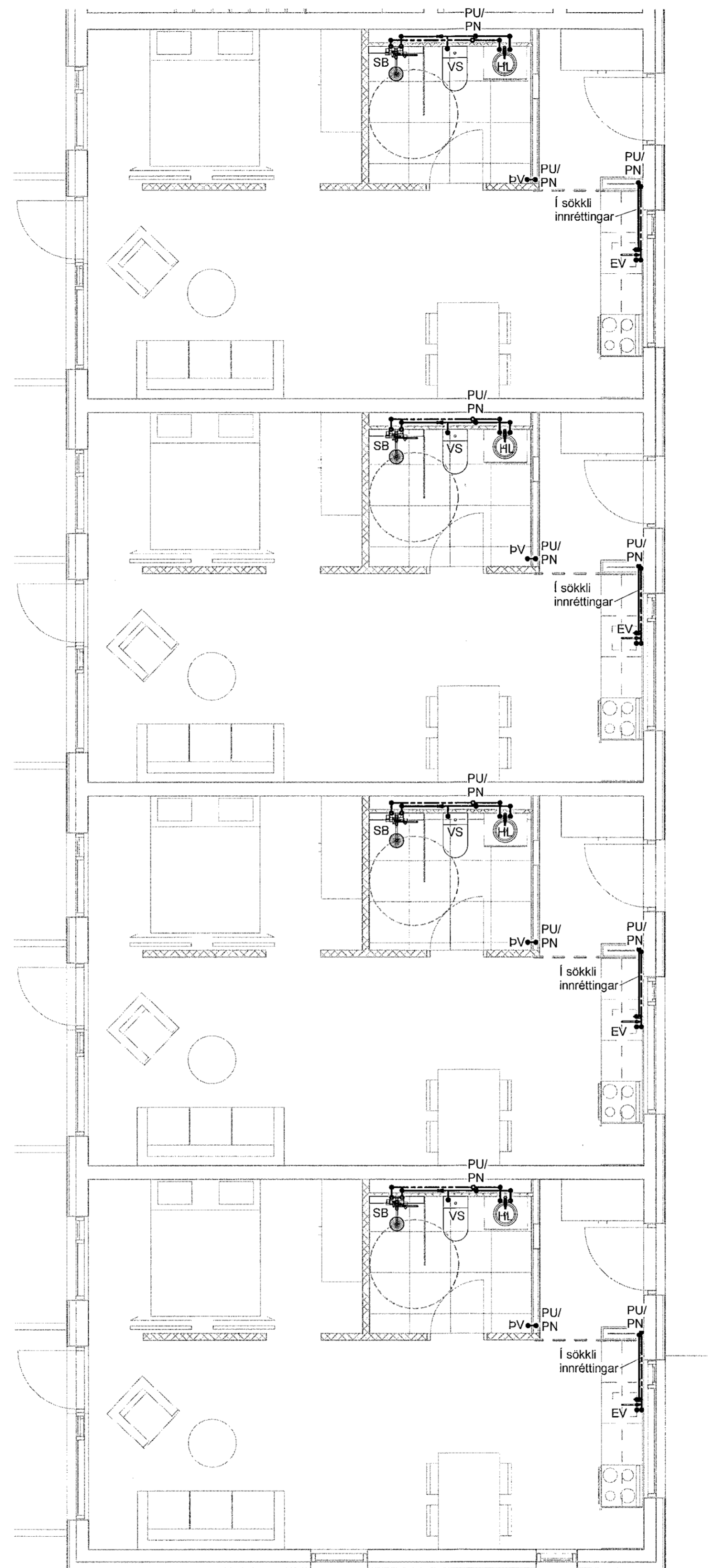
1 3. hæð - 1 1 : 50
