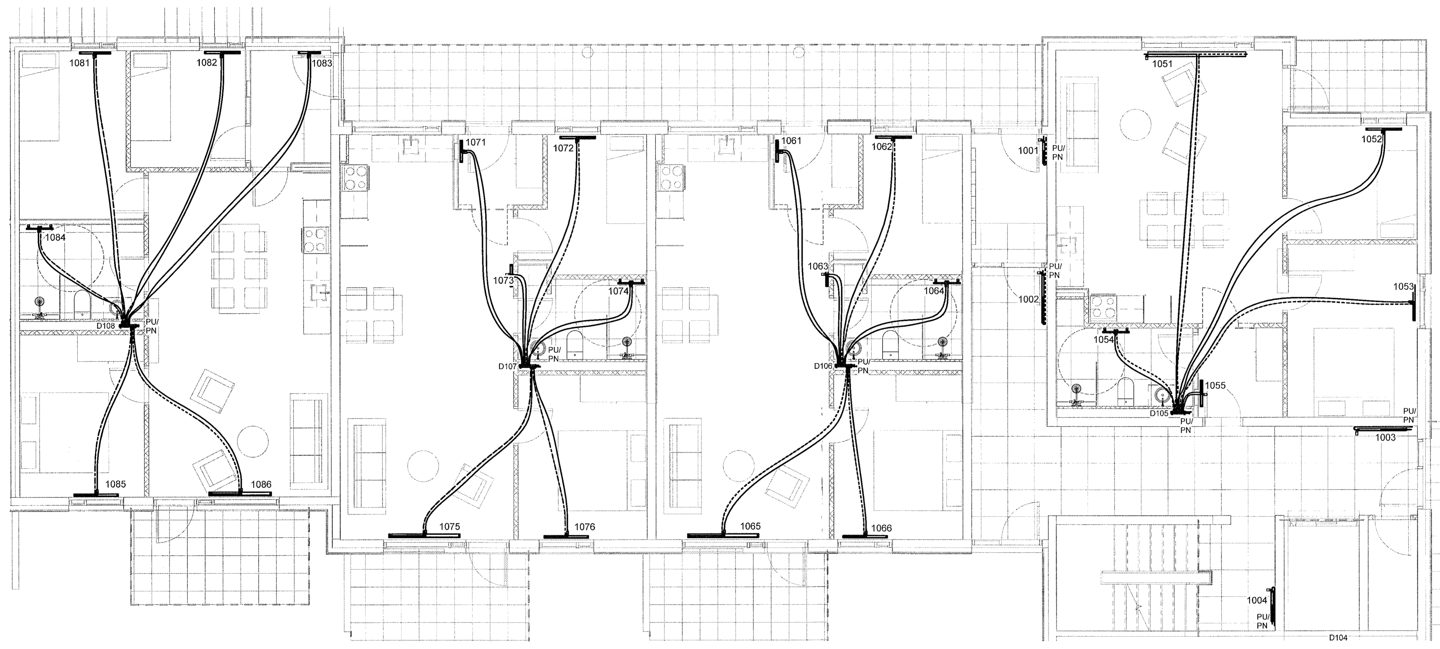
1 1.hæð - 2 1 : 50
