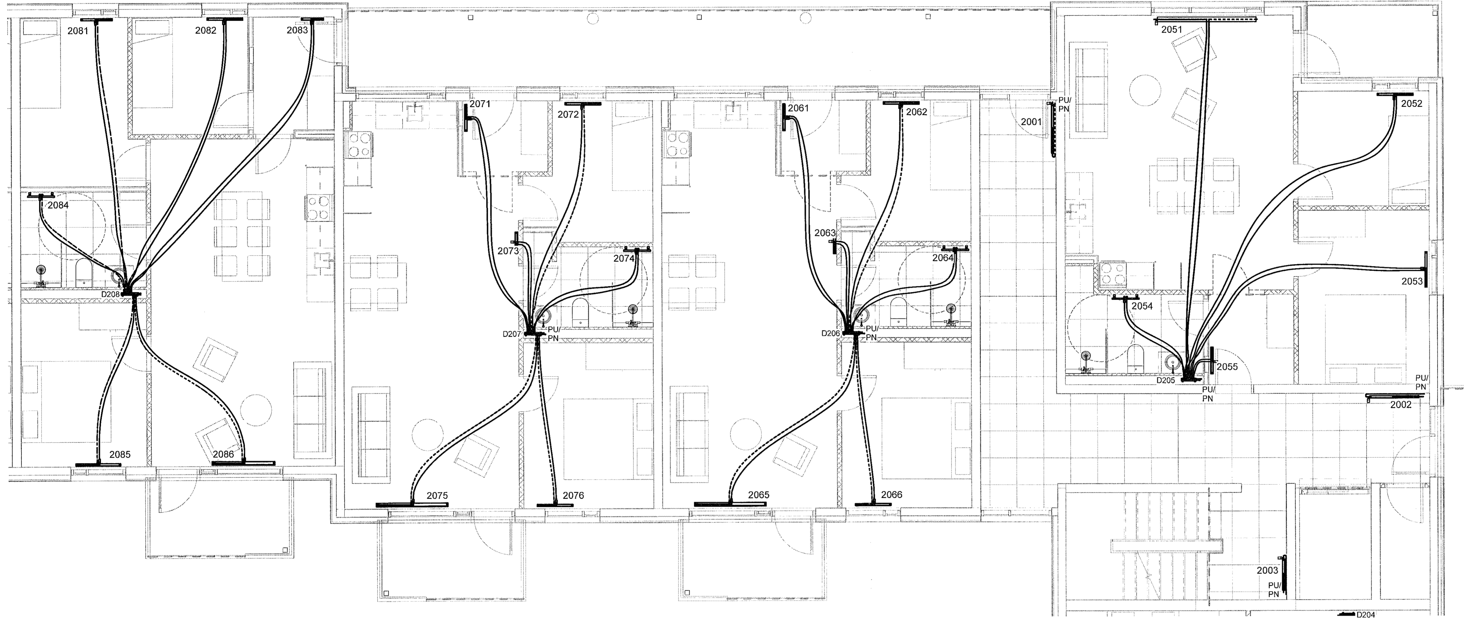
1 2. hæð - 2 1 : 50
