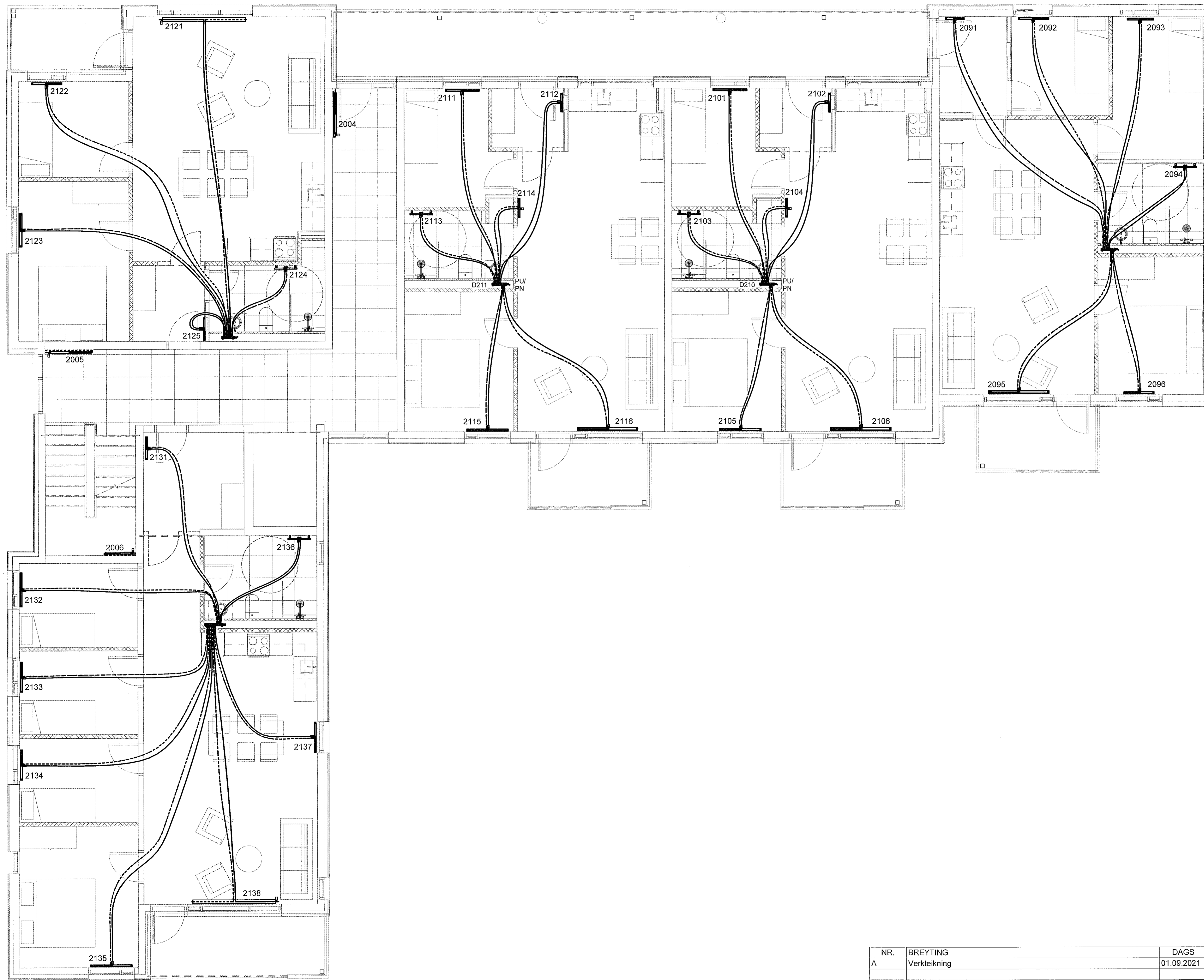
1 2. hæð - 3 1 : 50
