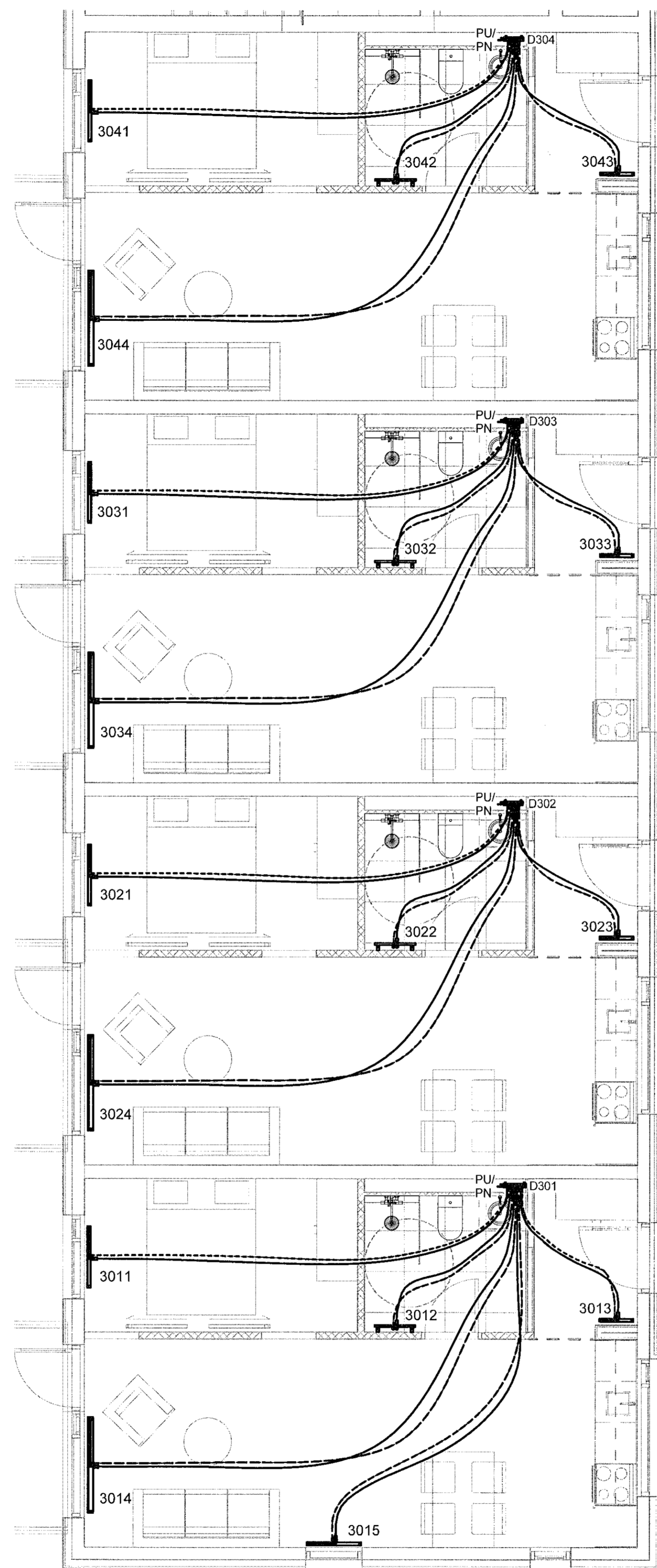
1 3. hæð - 2 1 : 50
