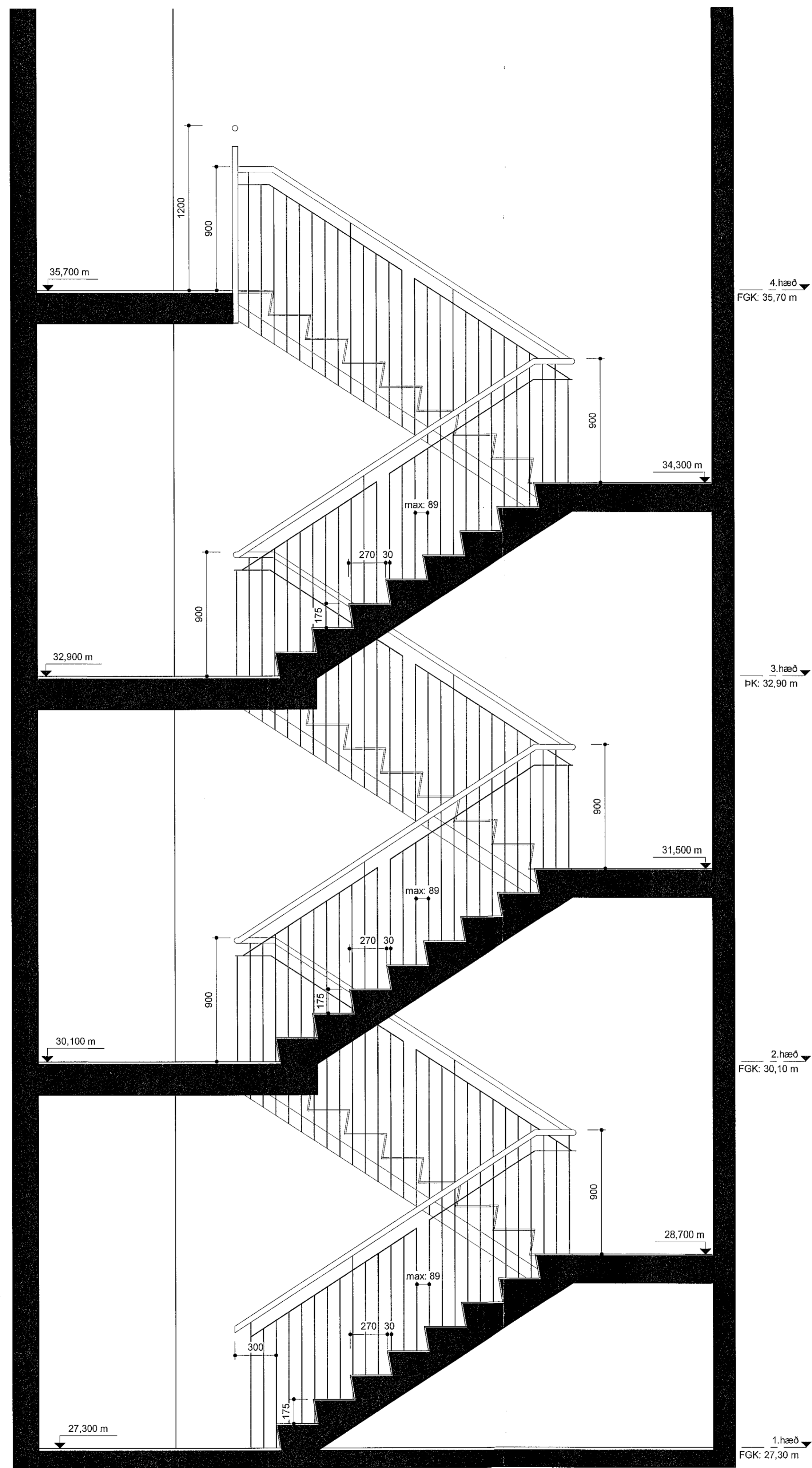
Stigi 2 - Snið 2-2
