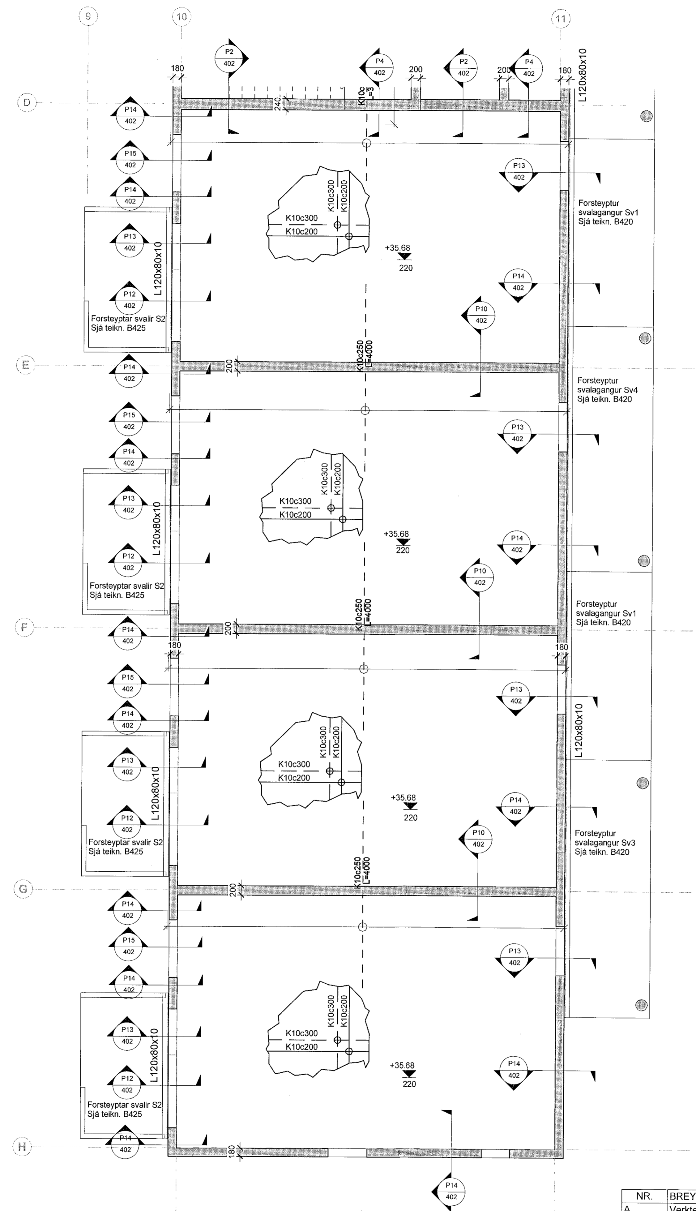
1 3. hæð - Loftaplata og veggir - 3/3 1 : 50
