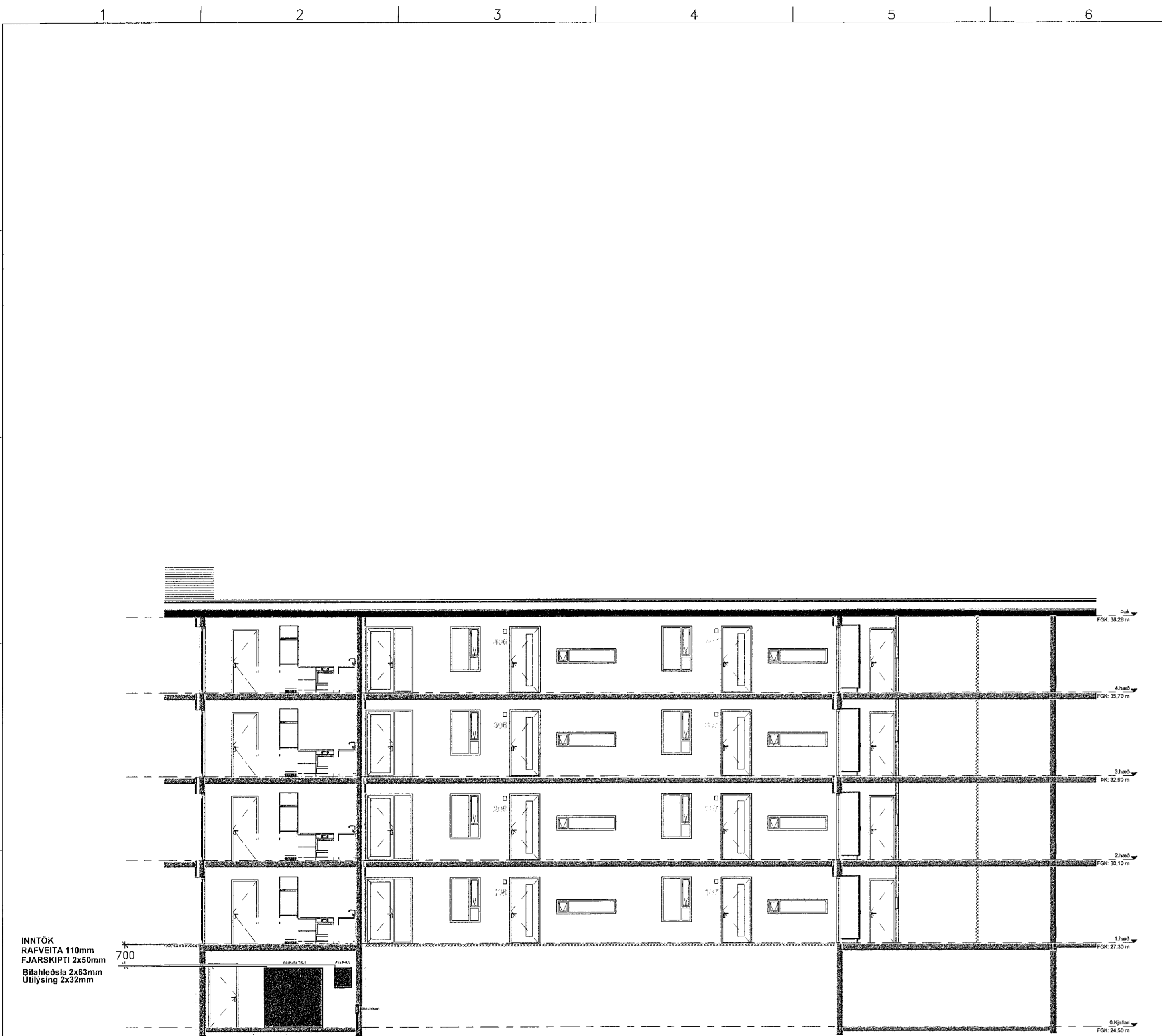
Sniðmynd 1:100
