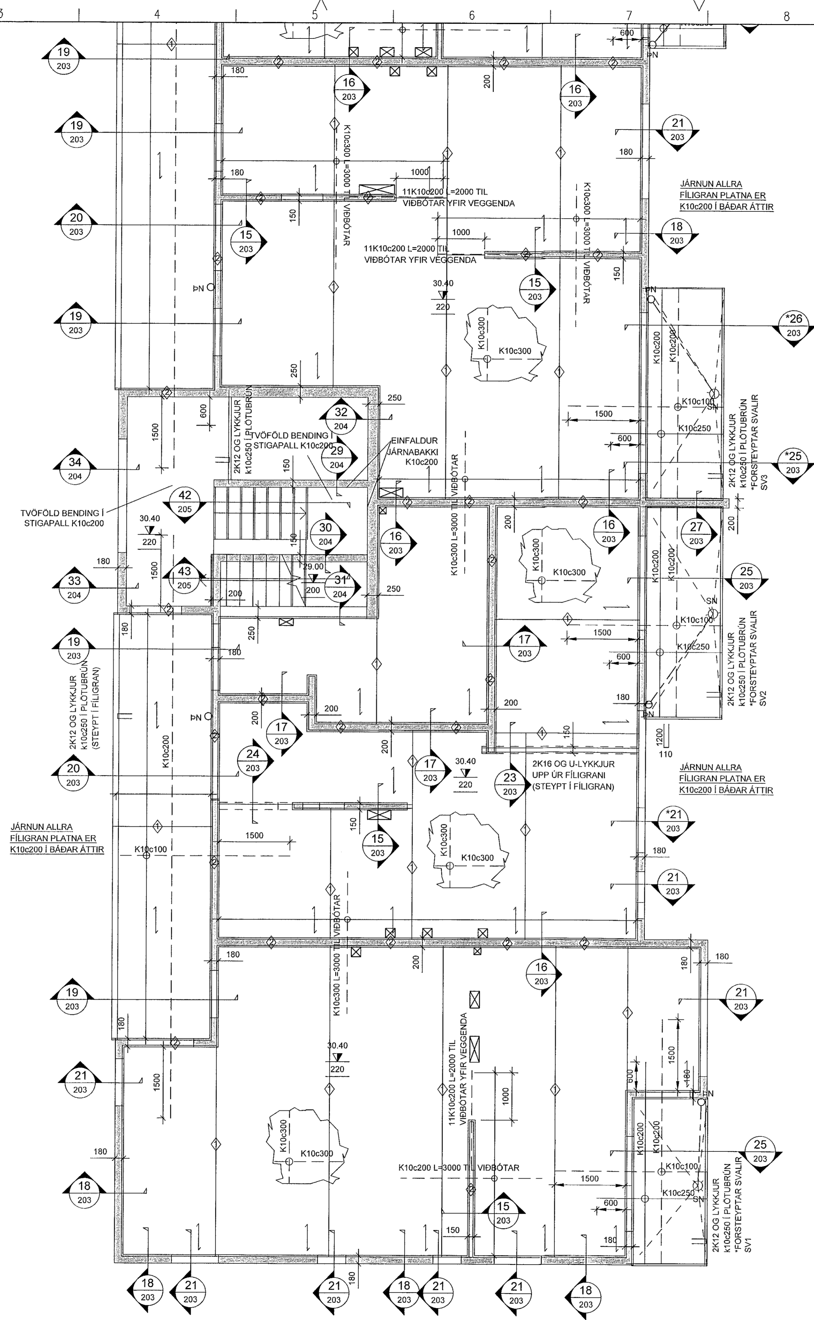
VEGGIR OG LOFTAPLATA 1.HÆÐAR, GRUNNMYND MKV. 3
