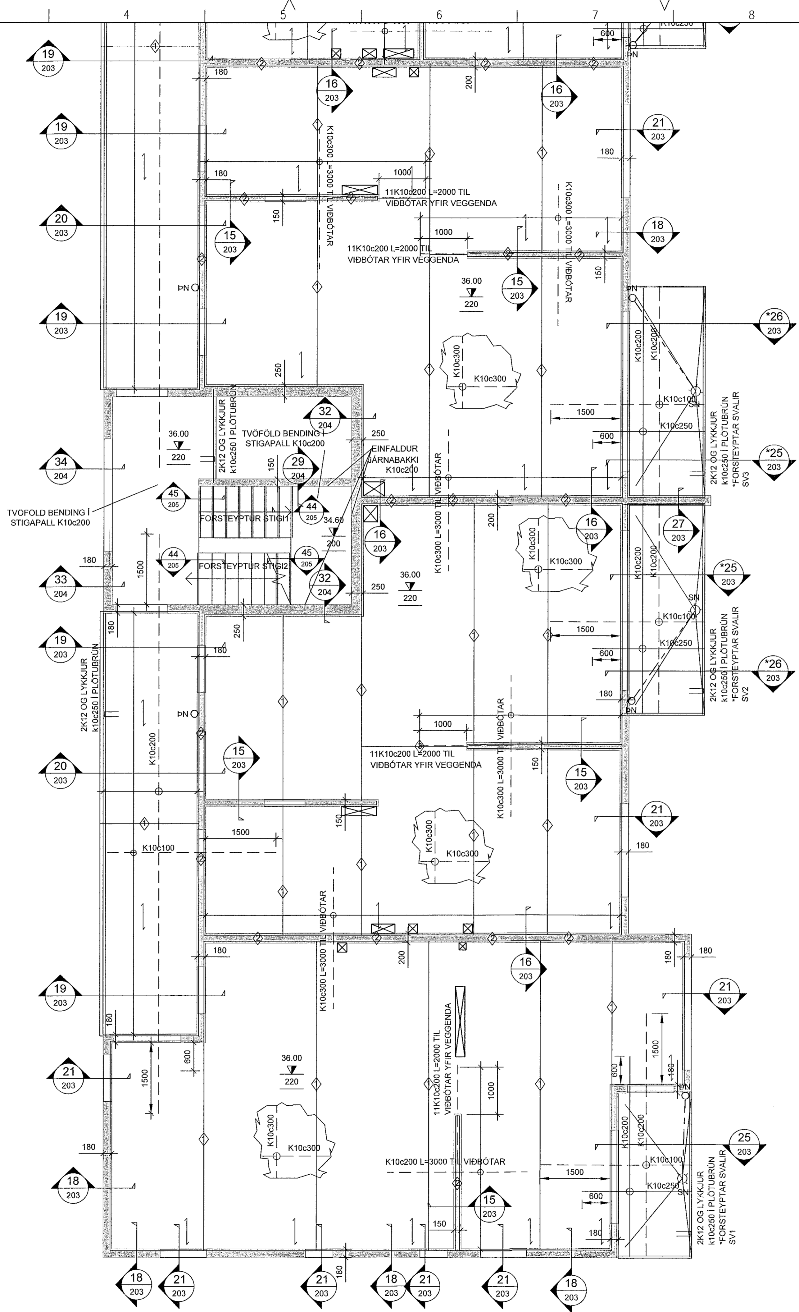
VEGGIR OG LOFTAPLATA 3.HÆÐAR, GRUNNMYND MKV. 3
