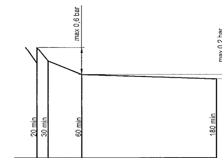
Þrýstiprófun á neysluvatnslögnum línurit
