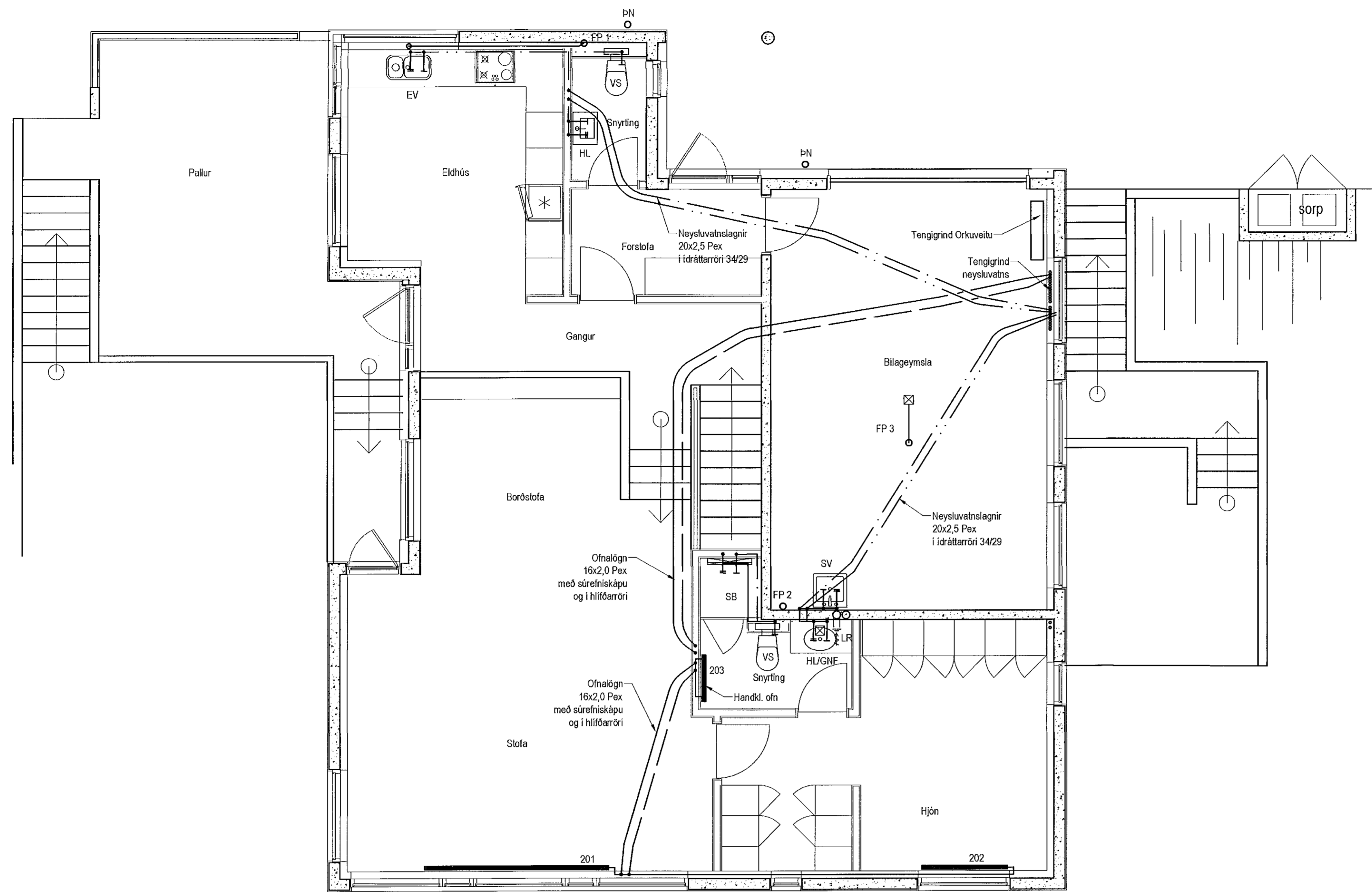
Neysluvatnslagnir 2. hæð, 1:50
