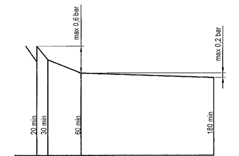
Þrýstifötun á neysluvatnslögnum línurit
