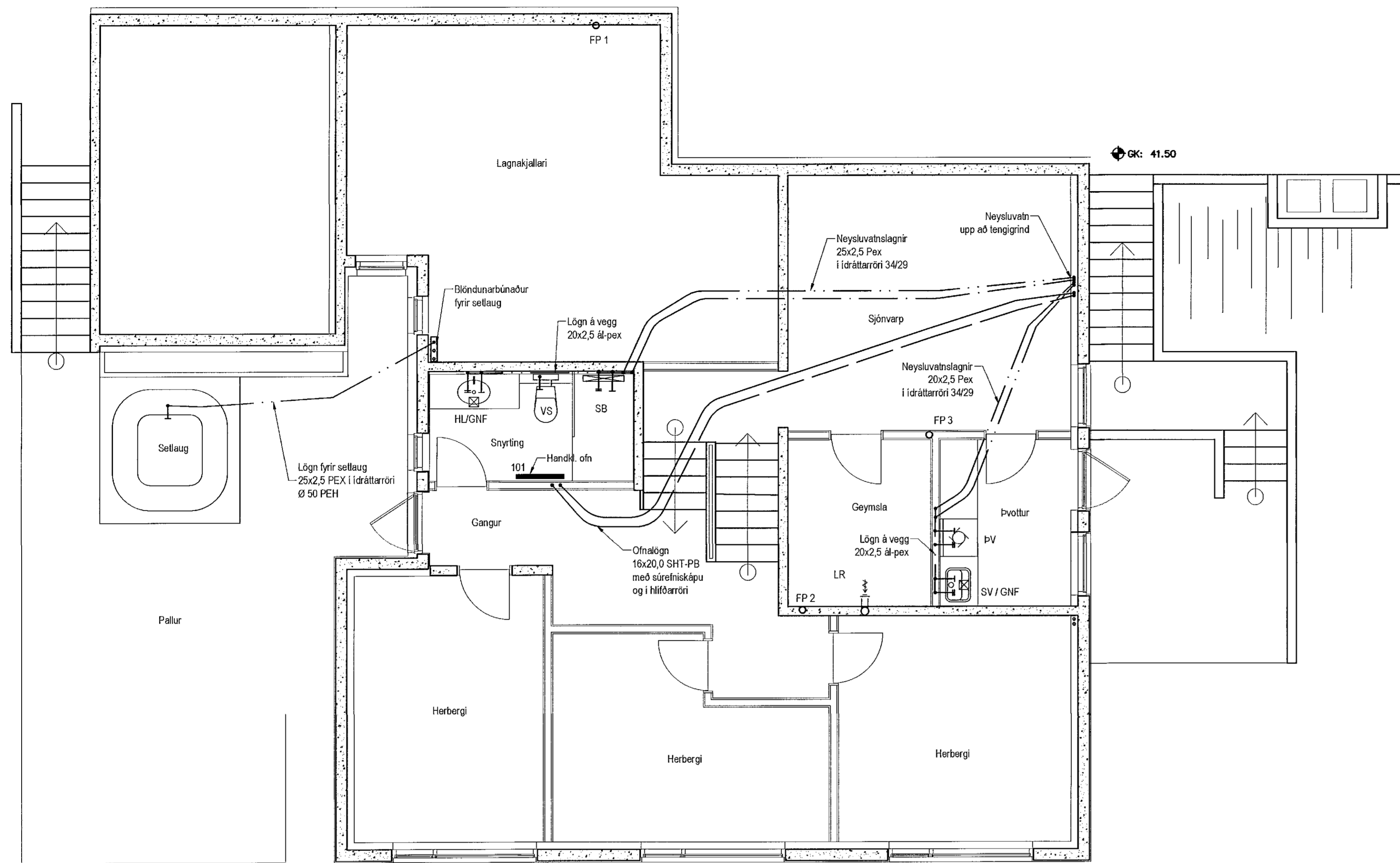
Neysluvatnslagnir 1. hæð, 1:50
