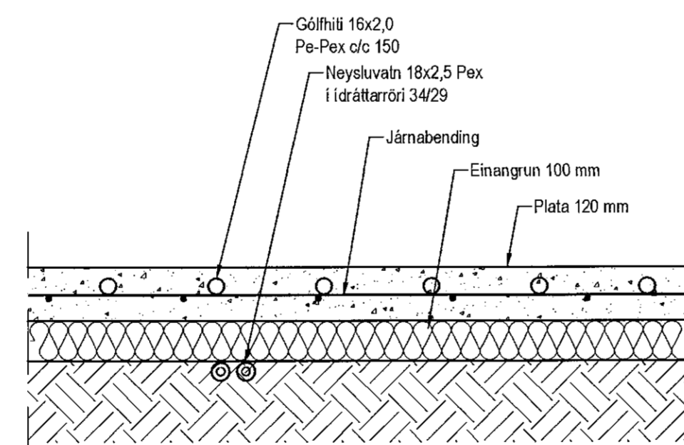
Hita- og vatnslagnir, Sníð í botnþötu, 1:10
