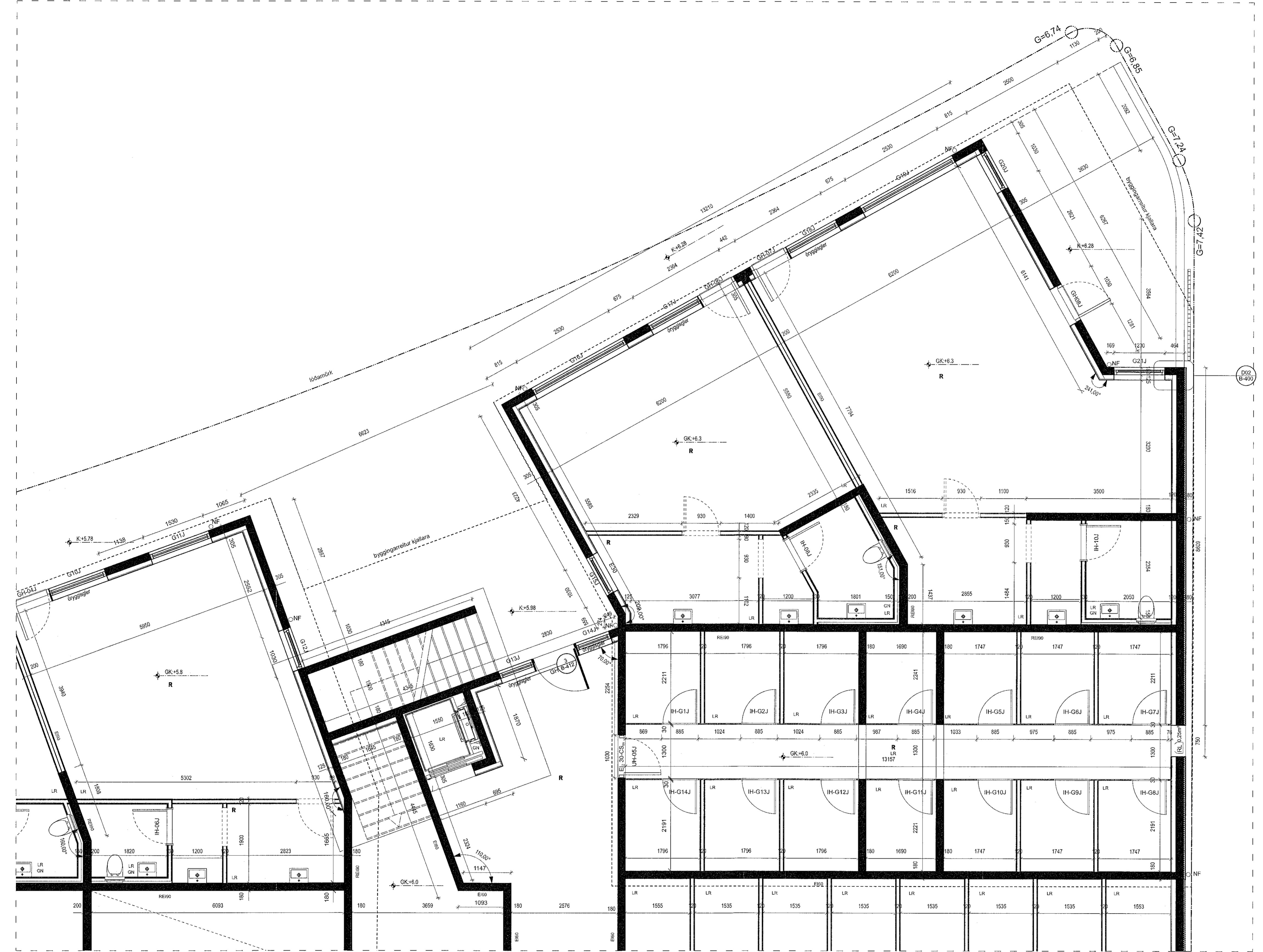
5 GRUNNMYND +1 Skali: 1:50
