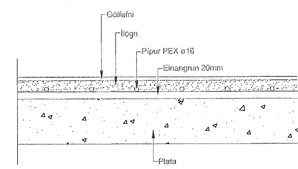
Snið í gólfhitalögn Pex ø16 M 1:10
