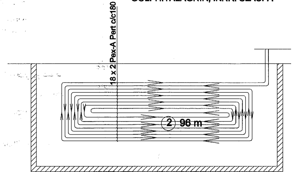
GÓLFHITALAGNIR, INNRI SLAUFU
