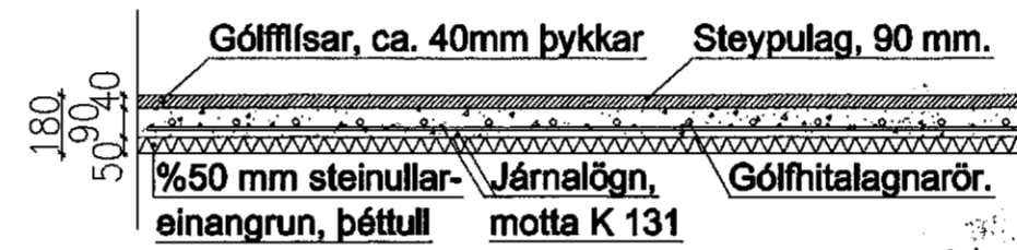
Gólf sólstofu, snið.
