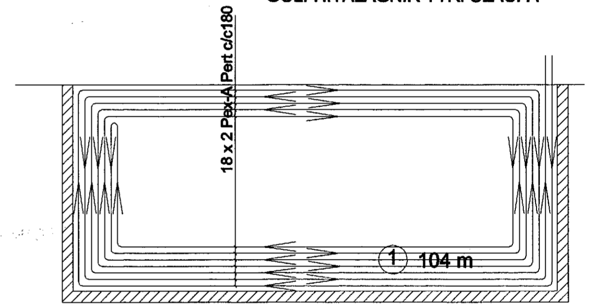
GÓLFHITALAGNIR YTRI SLAUFU
