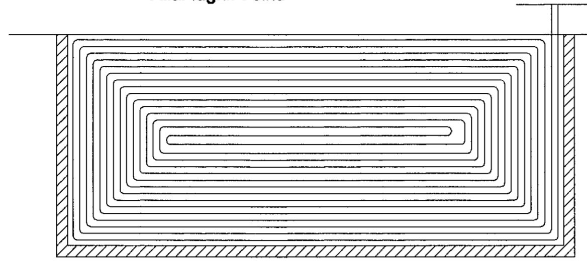
GÓLFHITALAGNIR Allar lagnir í einu
