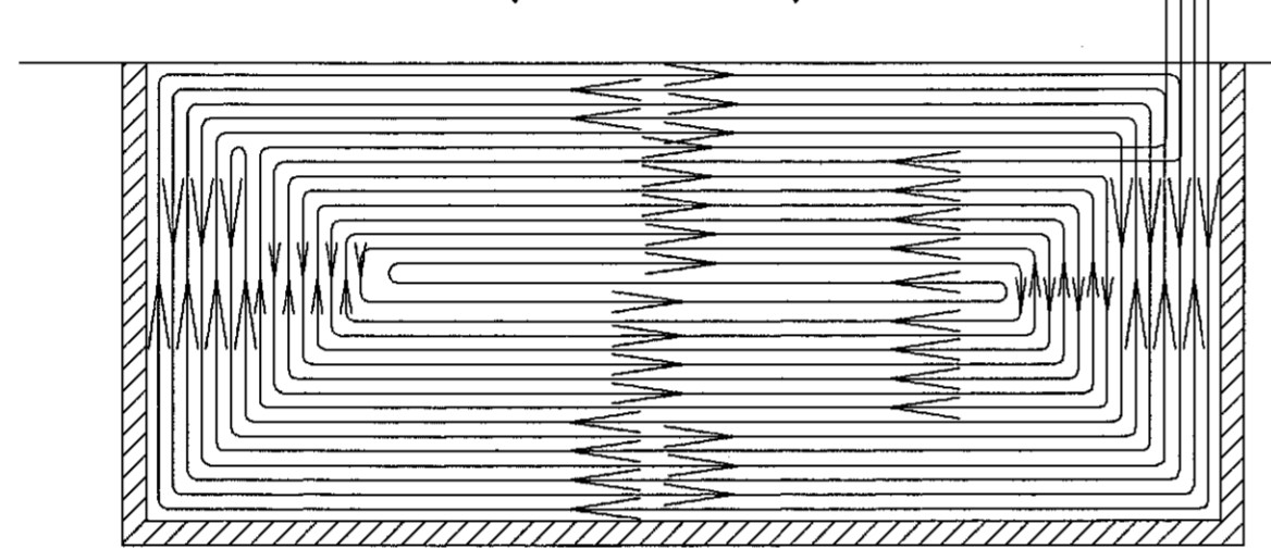
GÓLFHITALAGNIR, GRUNNMYND, BÁÐAR SLAUFUR.
