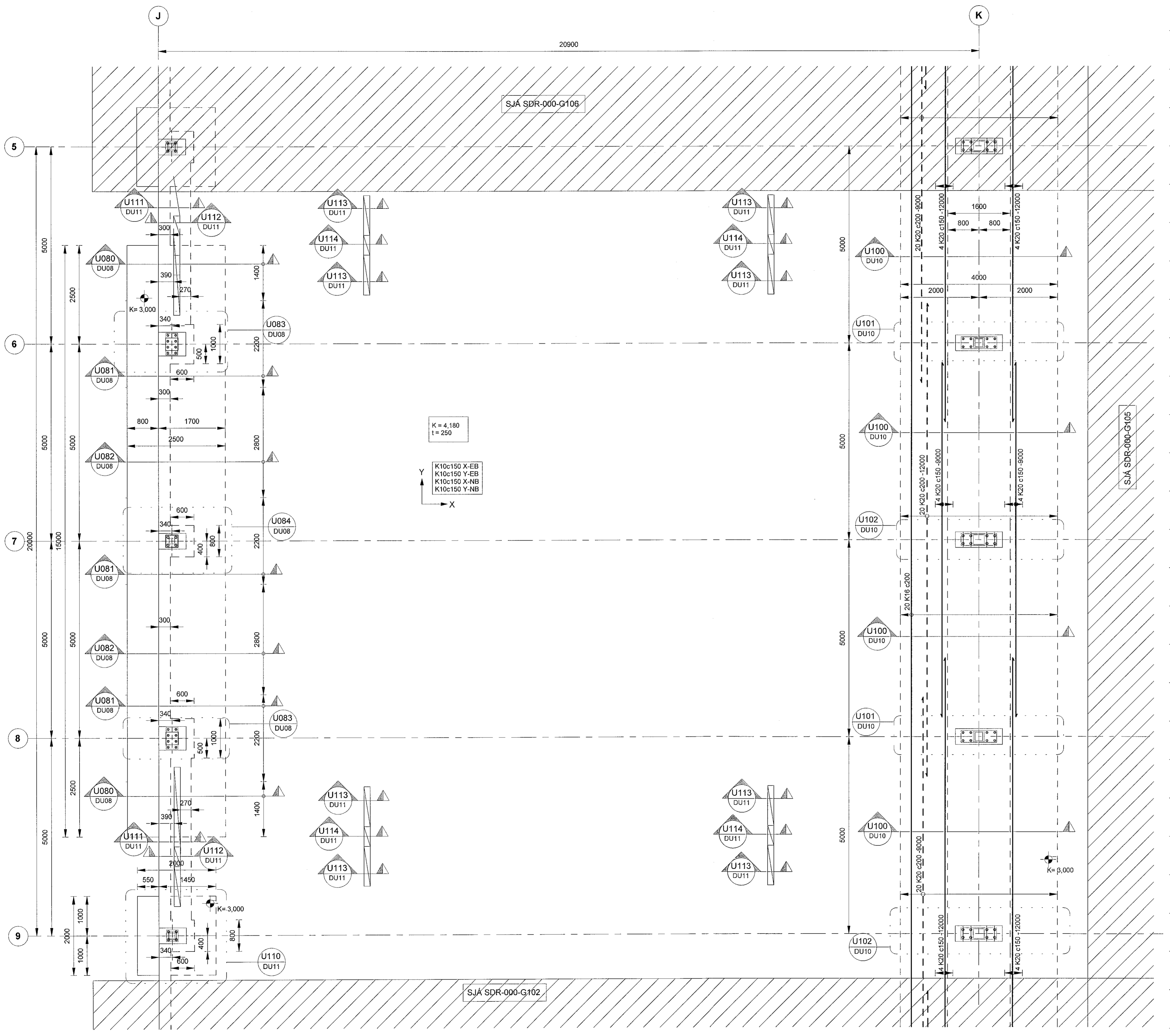
GRUNNMYND, HÆÐ 1. - HLUTI 4 1:50
