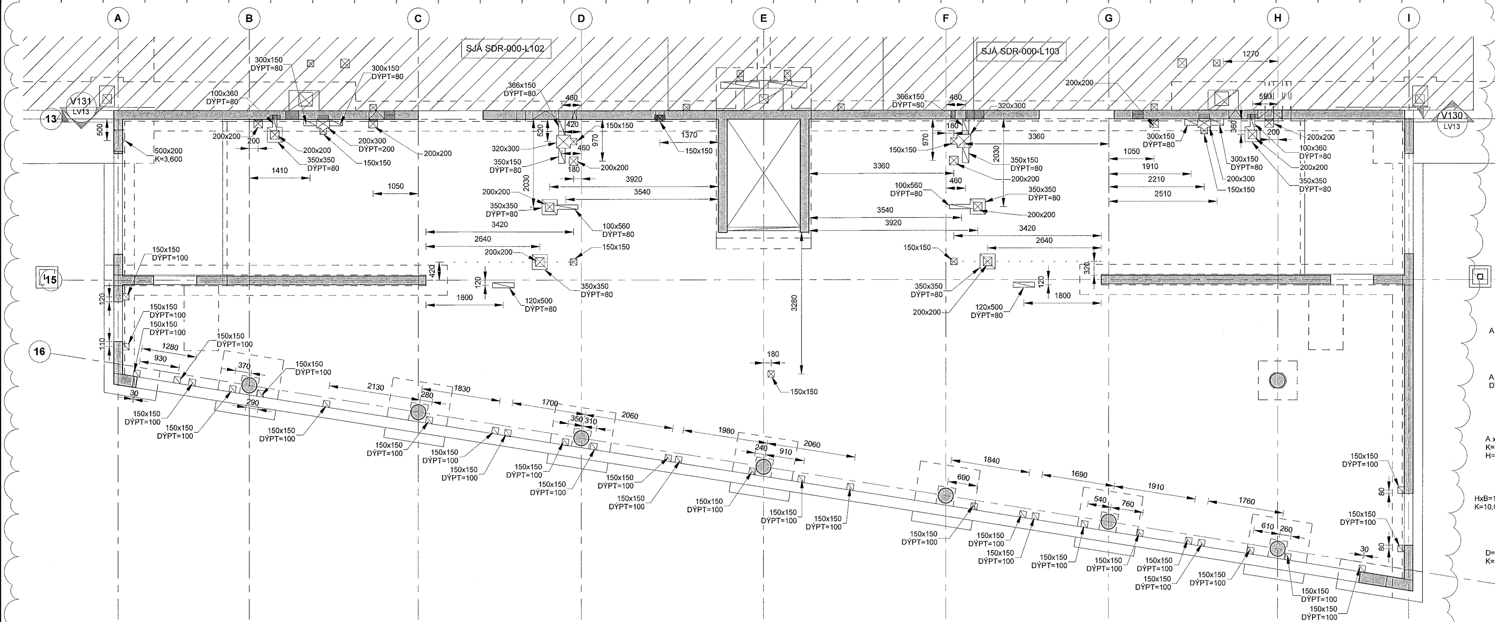
GRUNNMYND, HÆÐ 1, GATAPLAN - HLUTI 1 1:50
