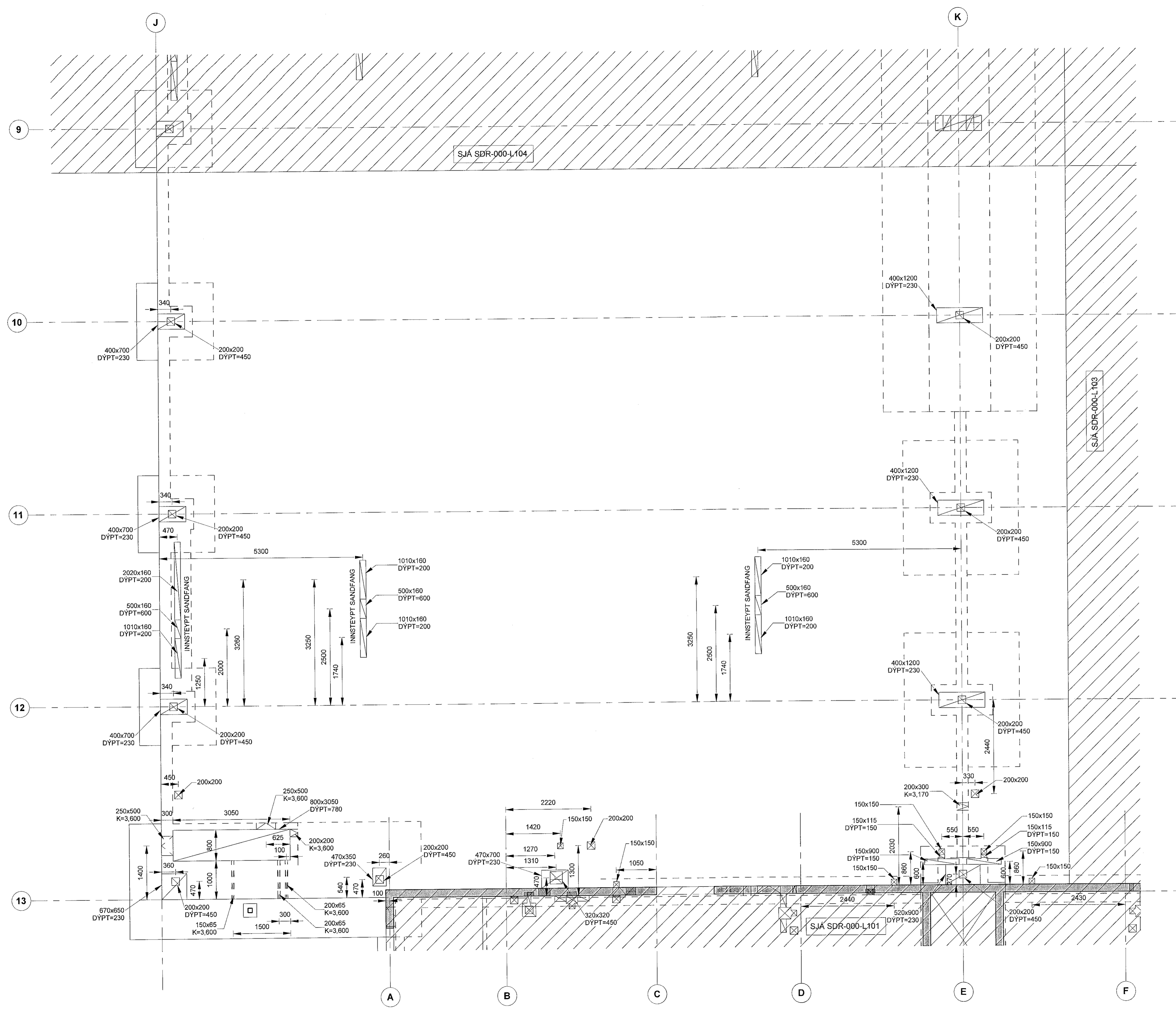
GRUNNMYND, HÆÐ 1, GATAPLAN - HLUTI 2 1:50
