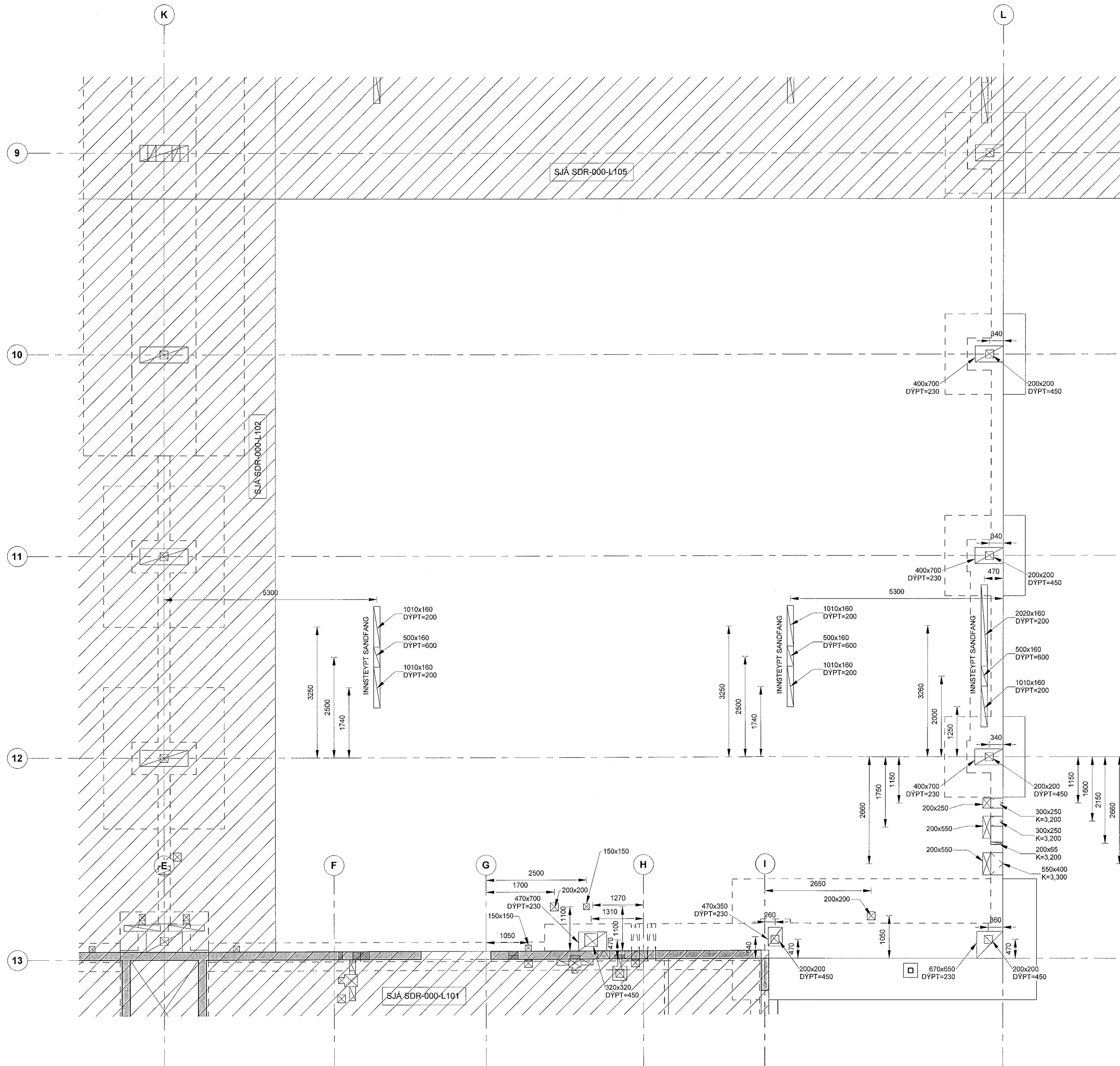
GRUNNMYND, HÆÐ 1, GATAPLAN - HLUTI 3 1:50
