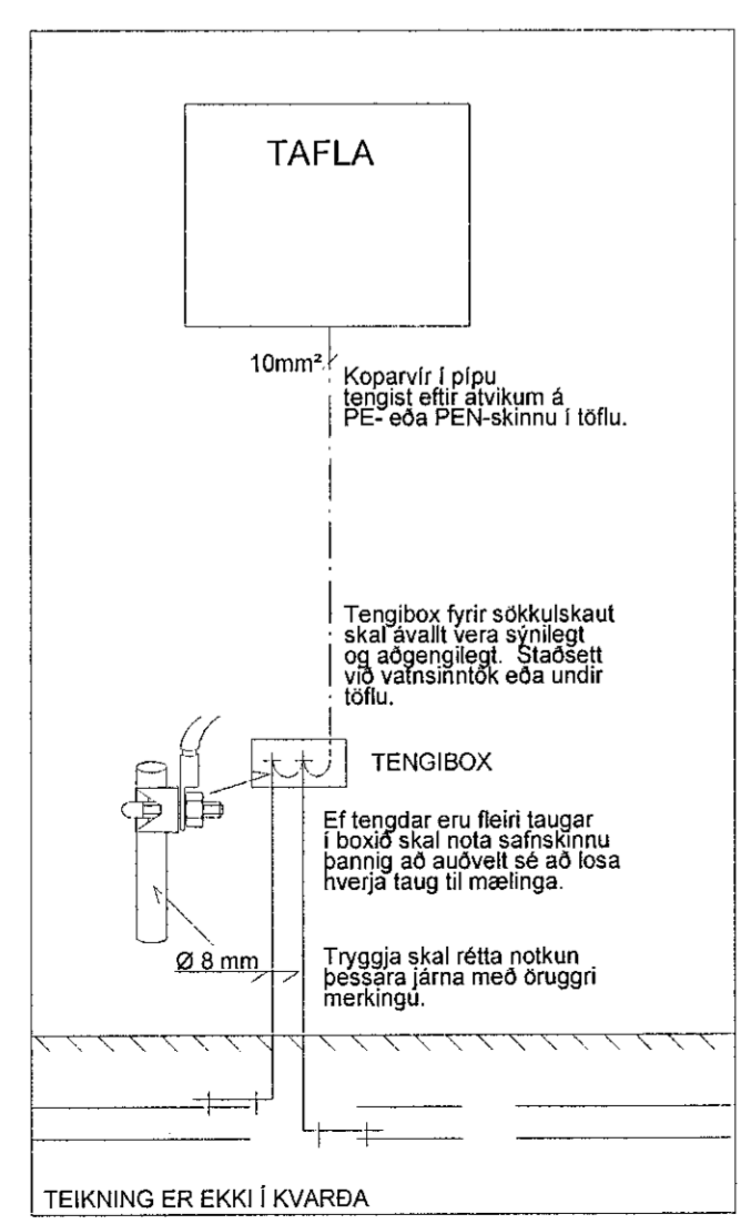
SNID Í TOFLUVEGG DÆMIGERÐUR FRÁGANGUR
