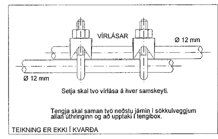
SAMTENGING STEYPUTEINA DÆMIGERÐUR FRÁGANGUR
