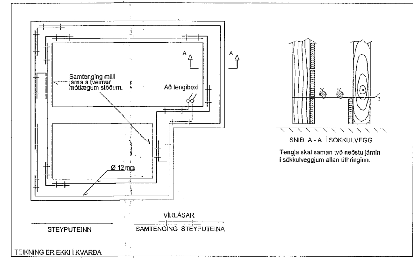
FYRIRMYND GRUNNMÝND SÖKKULVEGGJA DÆMIGERÐUR FRÁGANGUR
