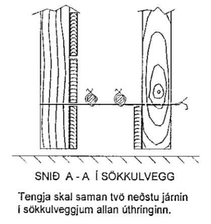
SNID A - A Í SÖKKULVEGG
