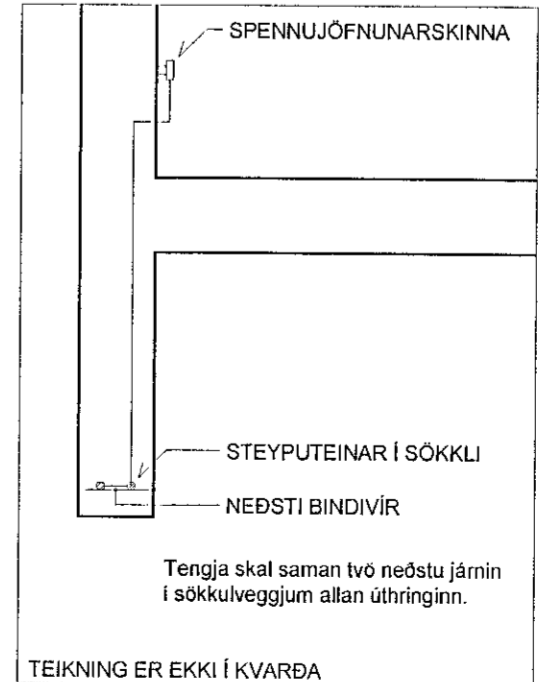
ÞVERSNÍÐ Í SÖKKLI DÆMIGERÐUR FRÁGANGUR
