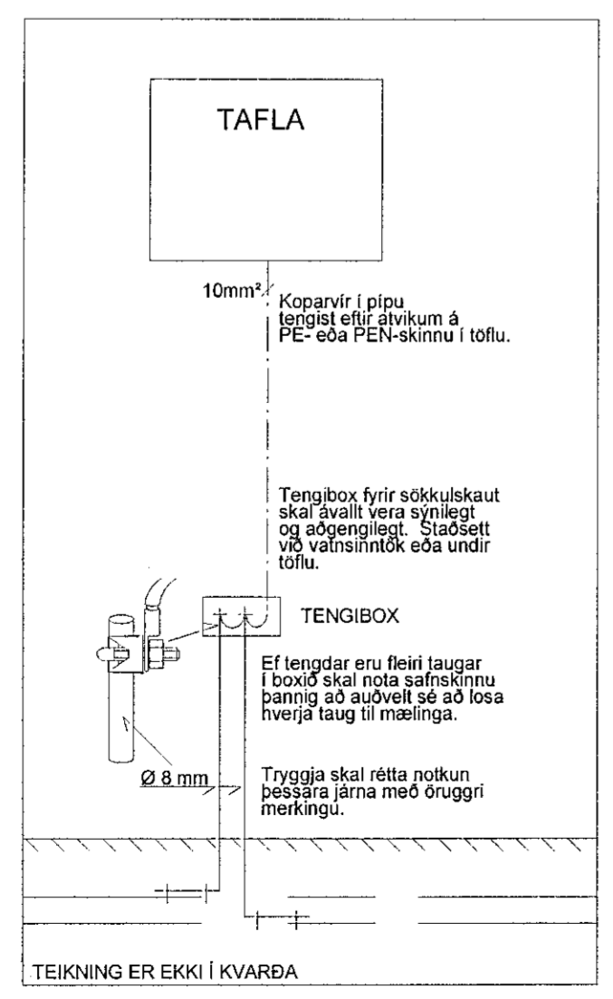
SNÍÐ Í TÖFLUVEGG DÆMIGERÐUR FRÁGANGUR
