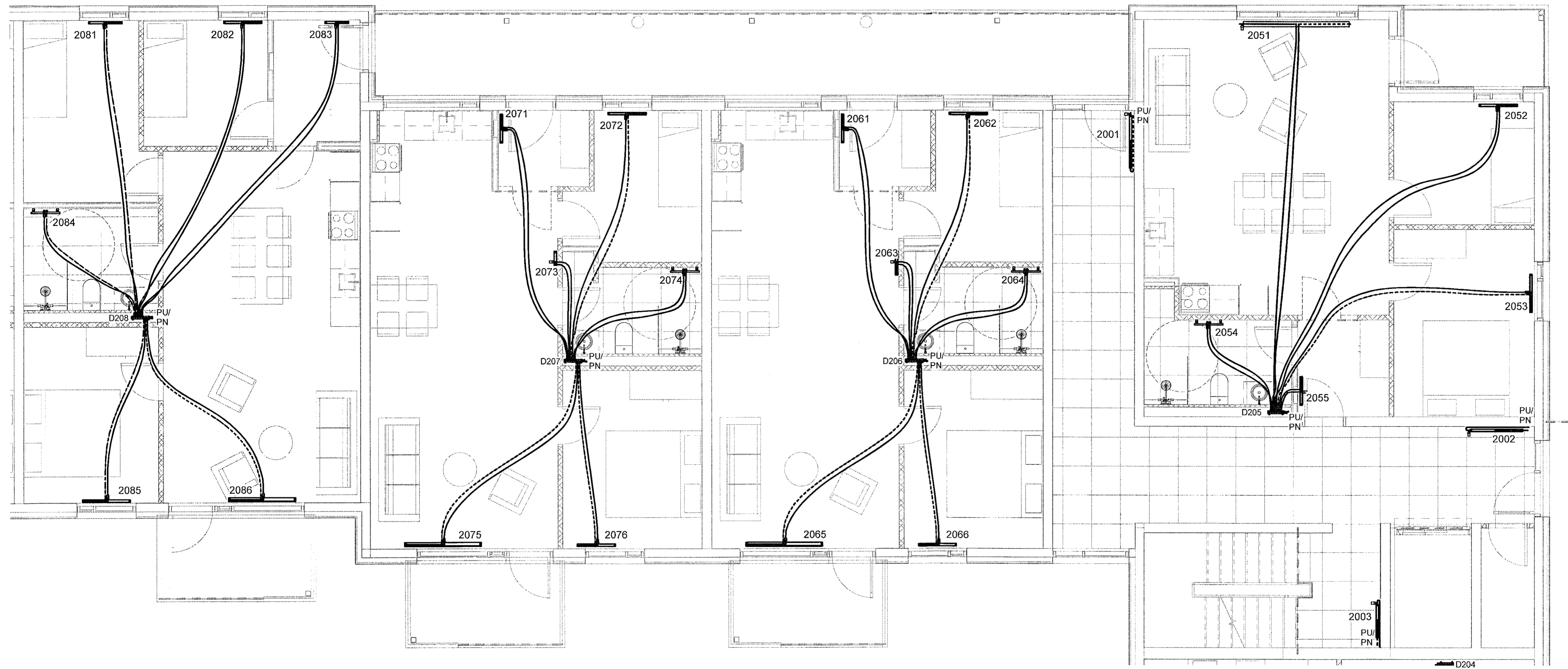
1 2. hæð - 2 1 : 50
