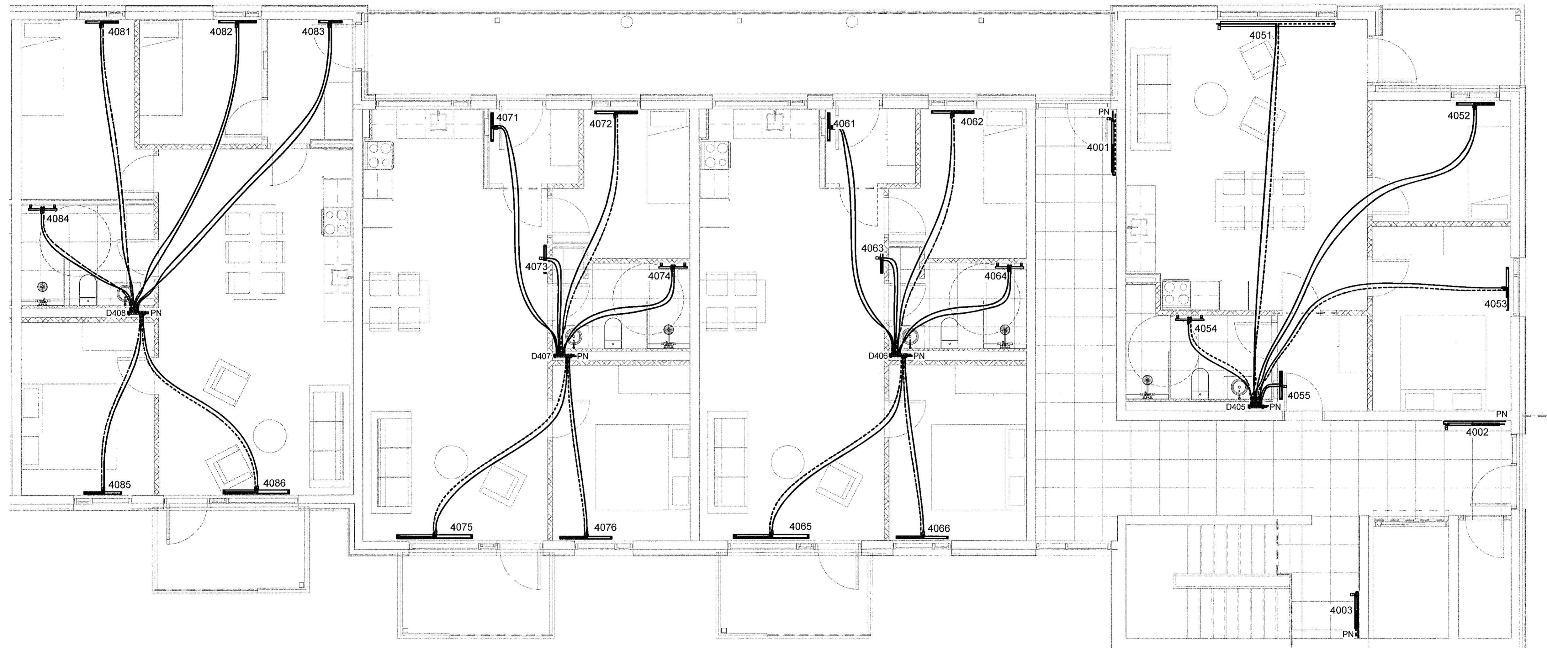
1 4. hæð - 2 1:50
