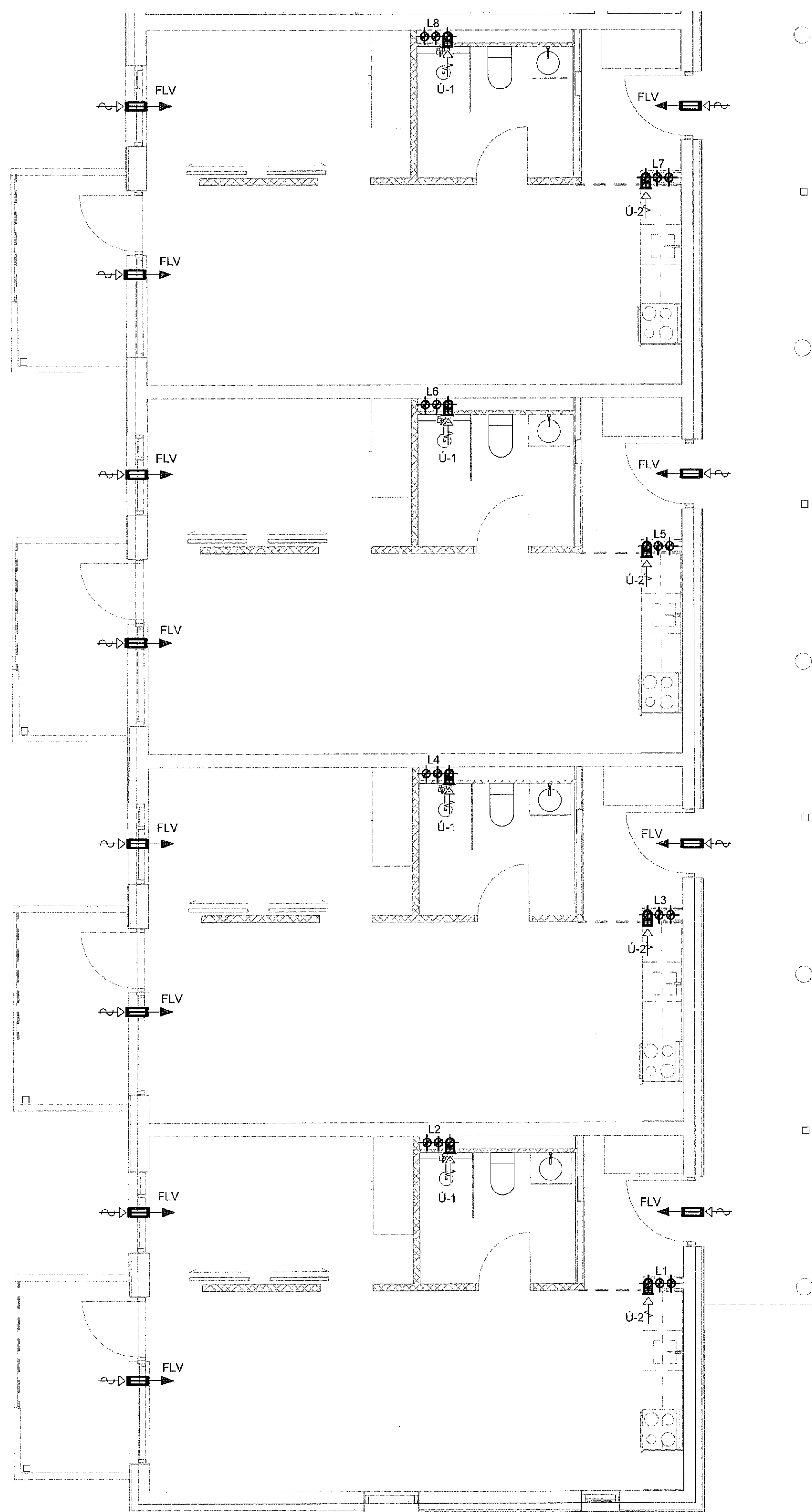
1 3. hæð - 1 1 : 50
