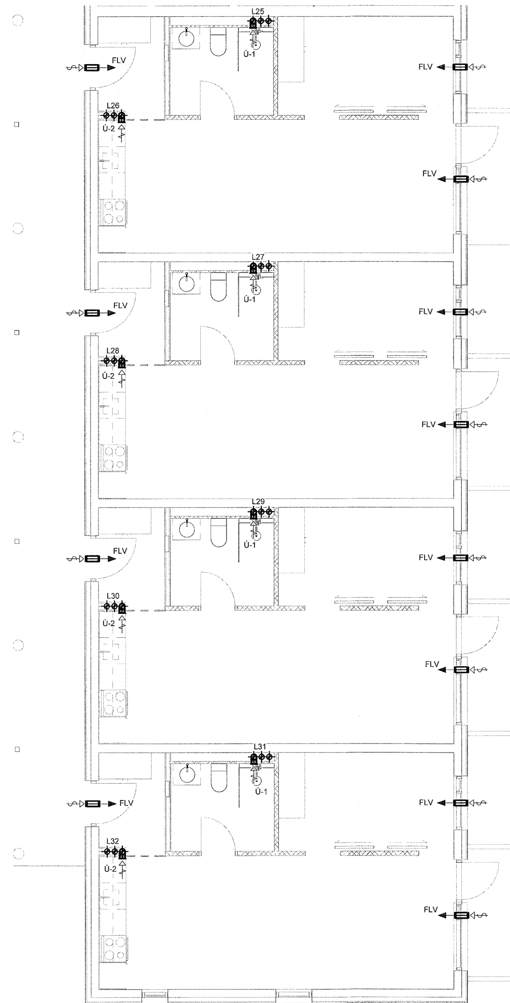
1 3. hæð - 4 1 : 50
