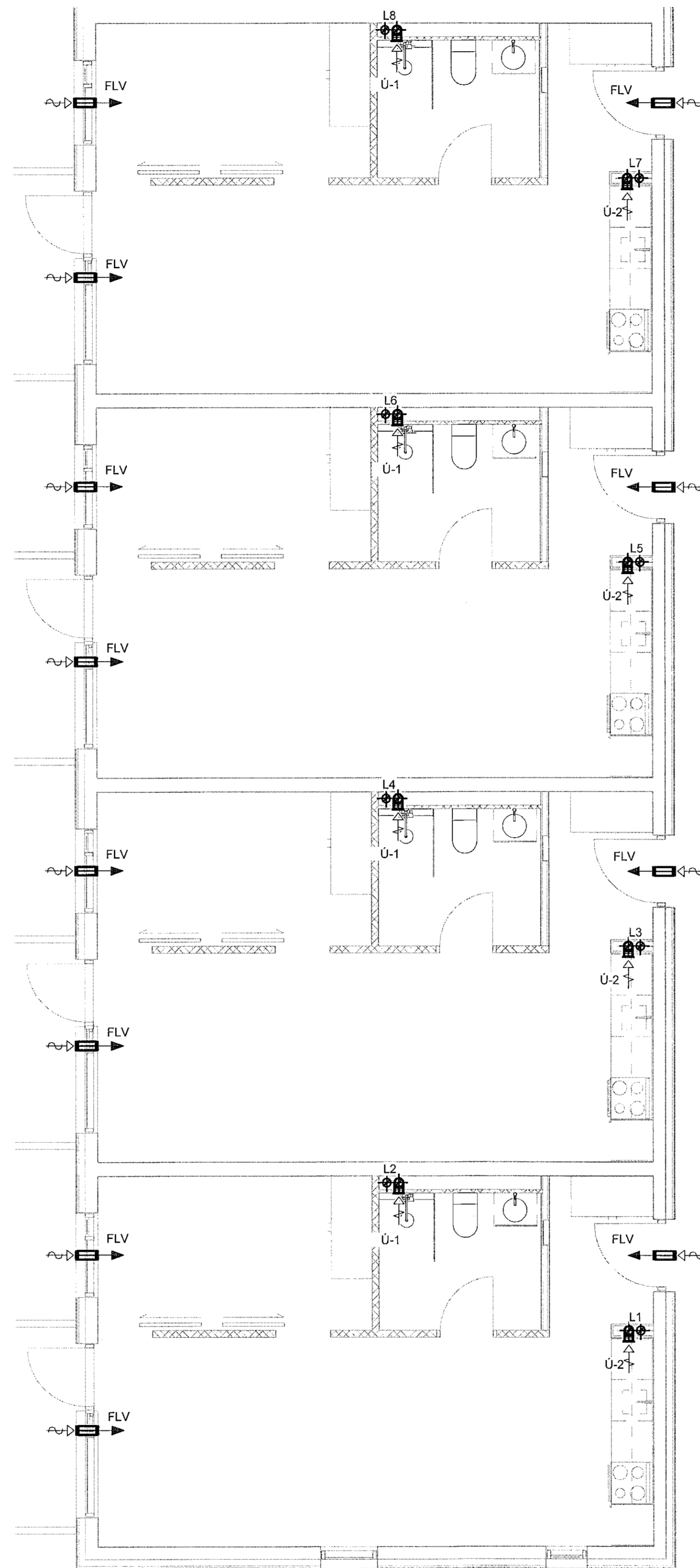
1 2. hæð - 1 1 : 50
