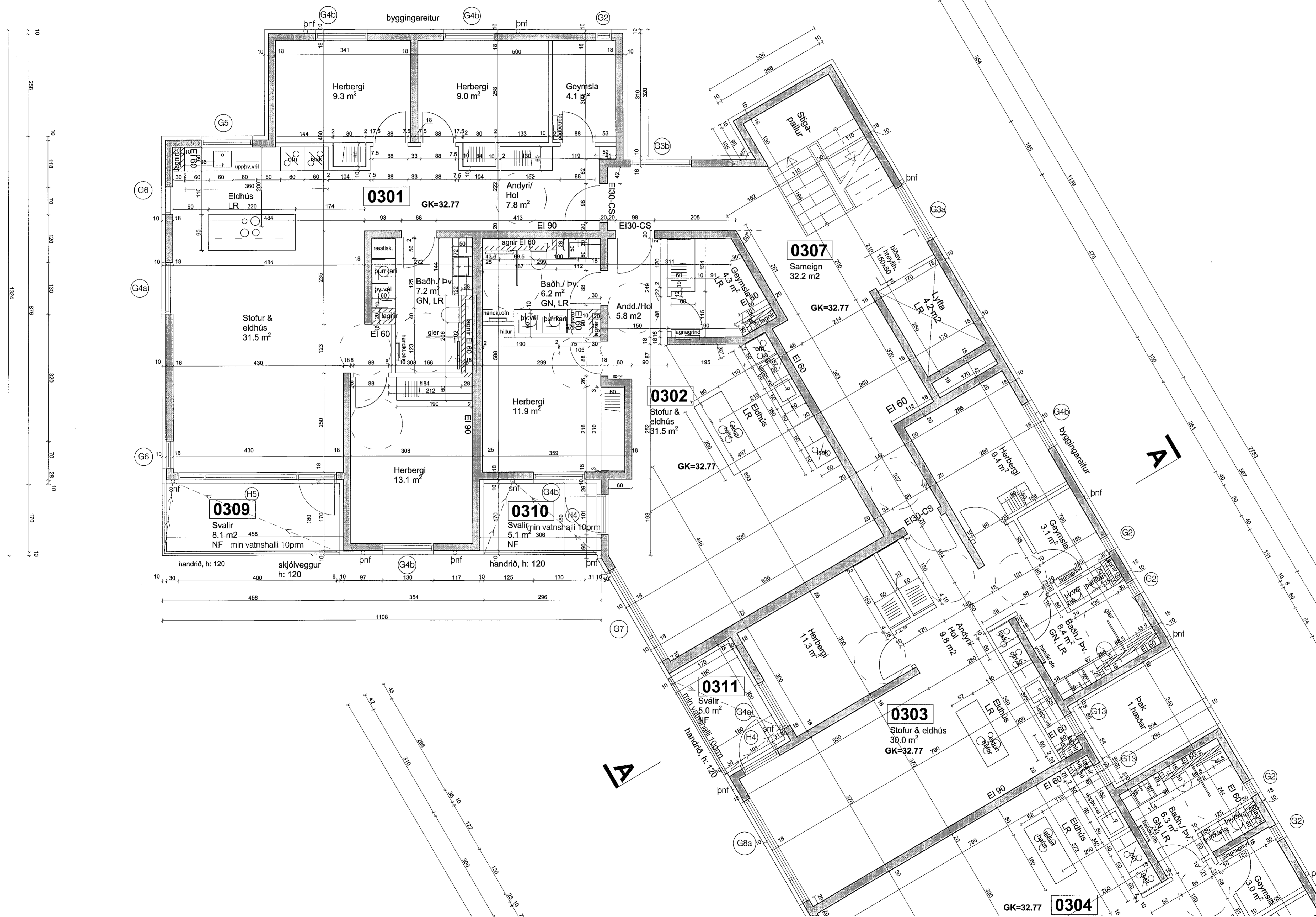
Grunnmynd 3.hæð, Nónhamar 2
