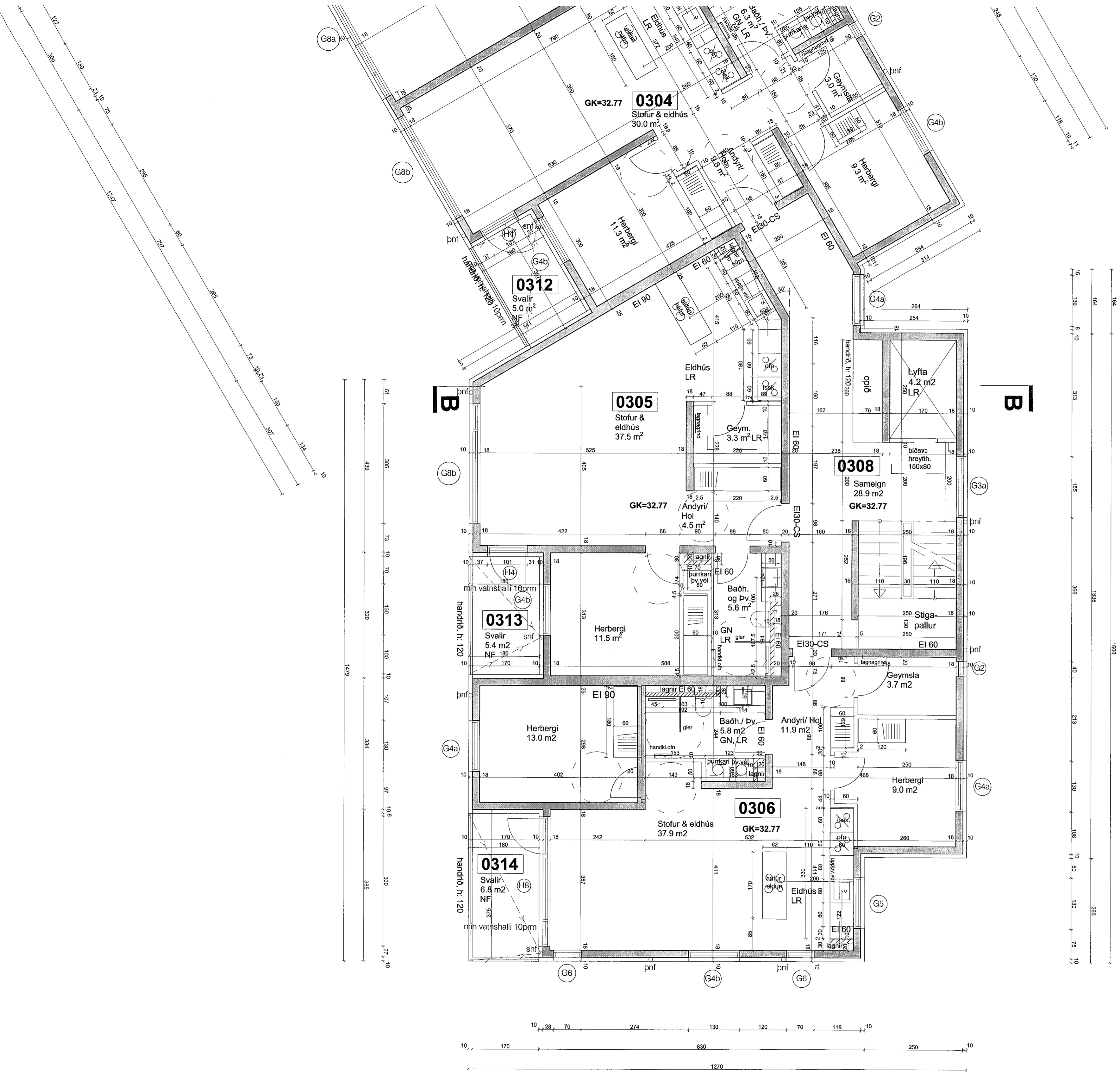
Grunnmynd 3.hæð, Nónhamar 2
