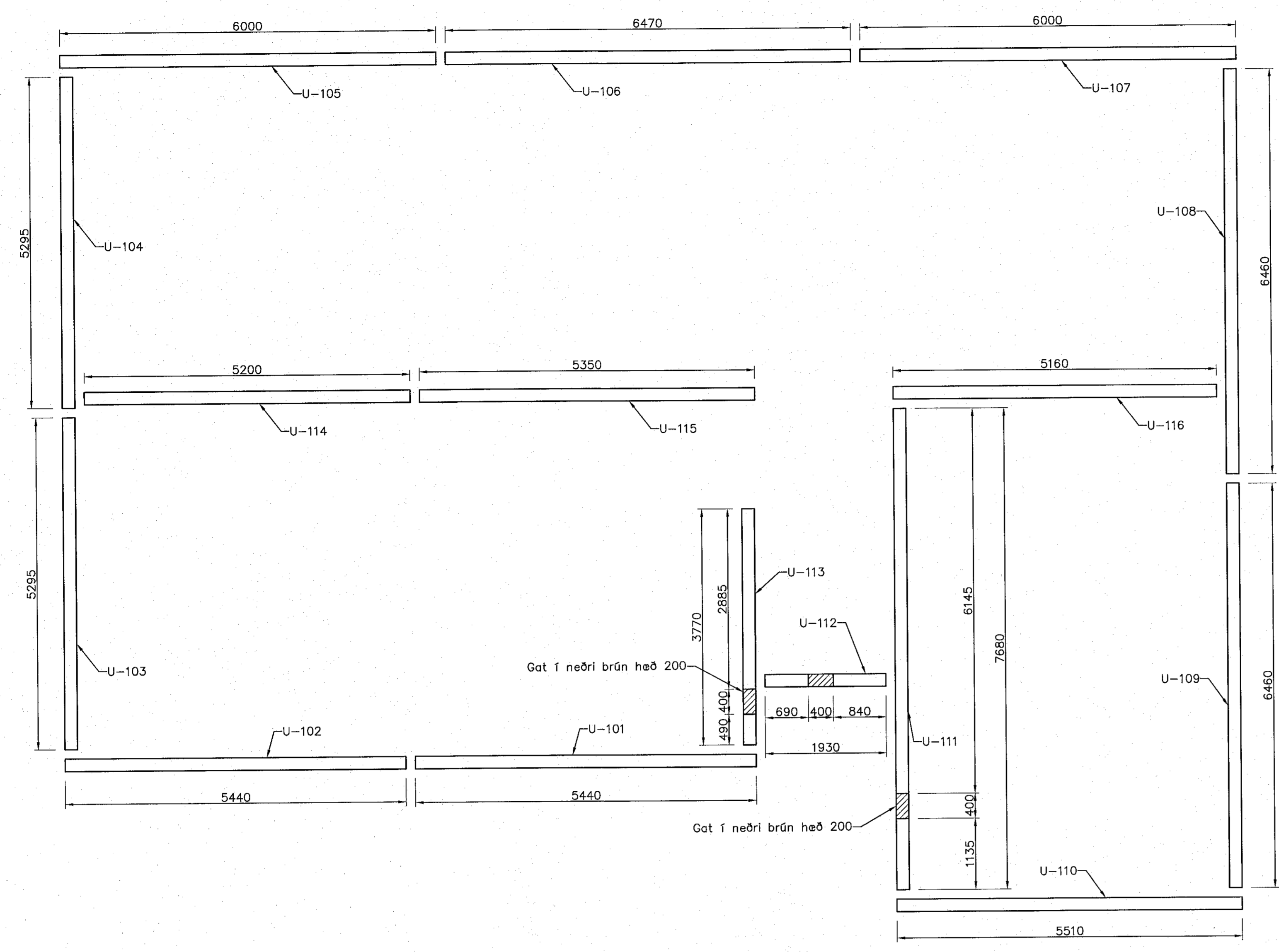
Undirstöður einingar, Grunnmynd, 1:50
