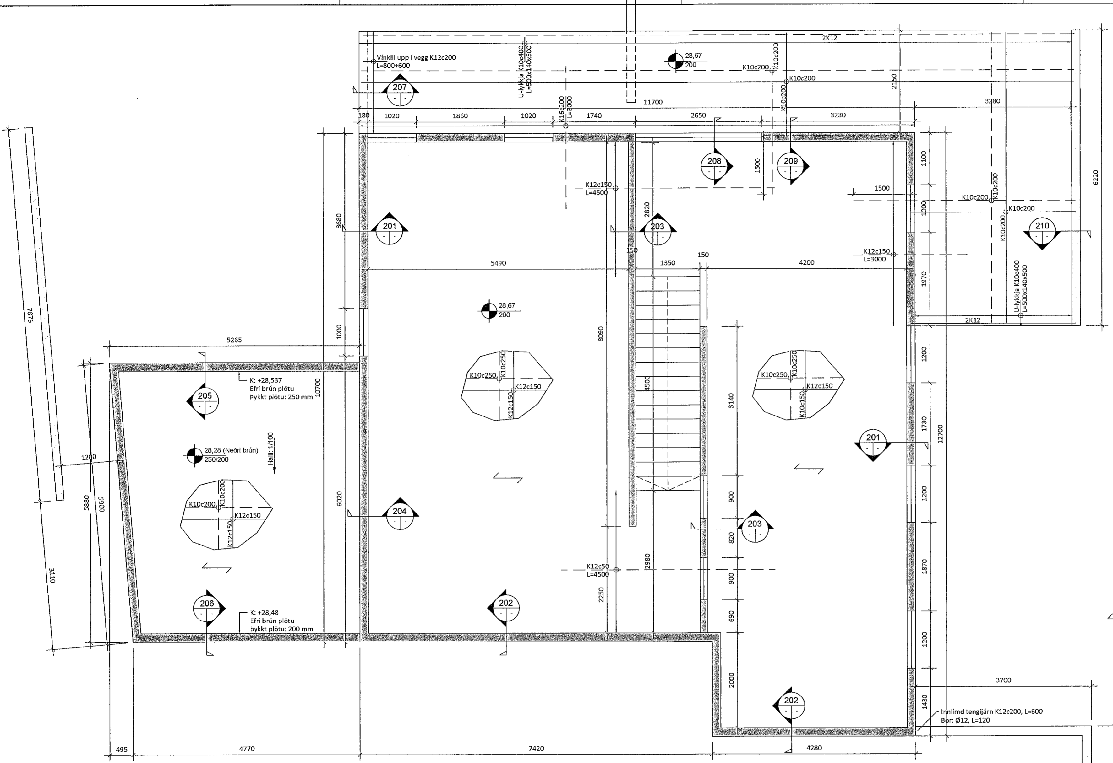
Grunnmynd - Plata yfir 1. hæð Mkv. 1:50
