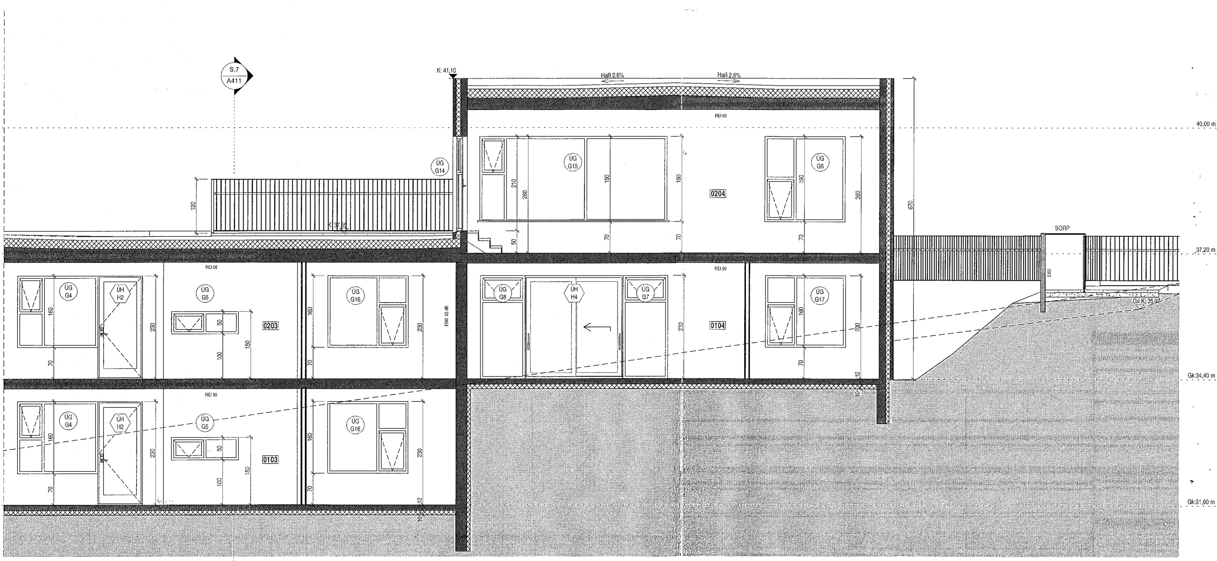
Snið 2b 1:50
