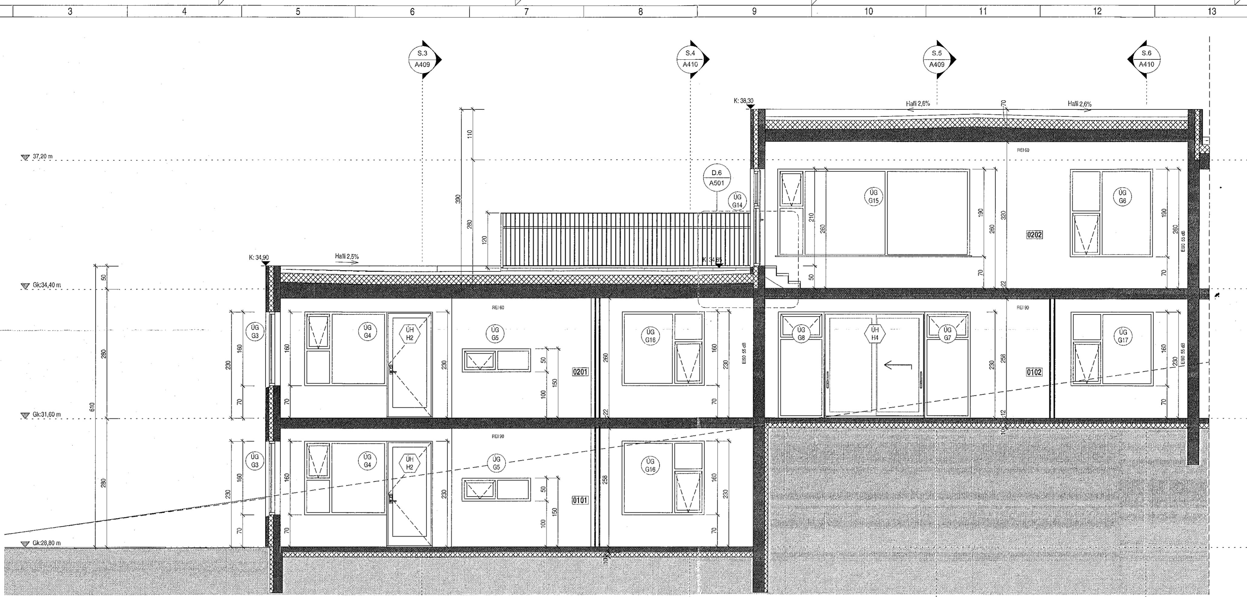
Snið 2a 1:50
