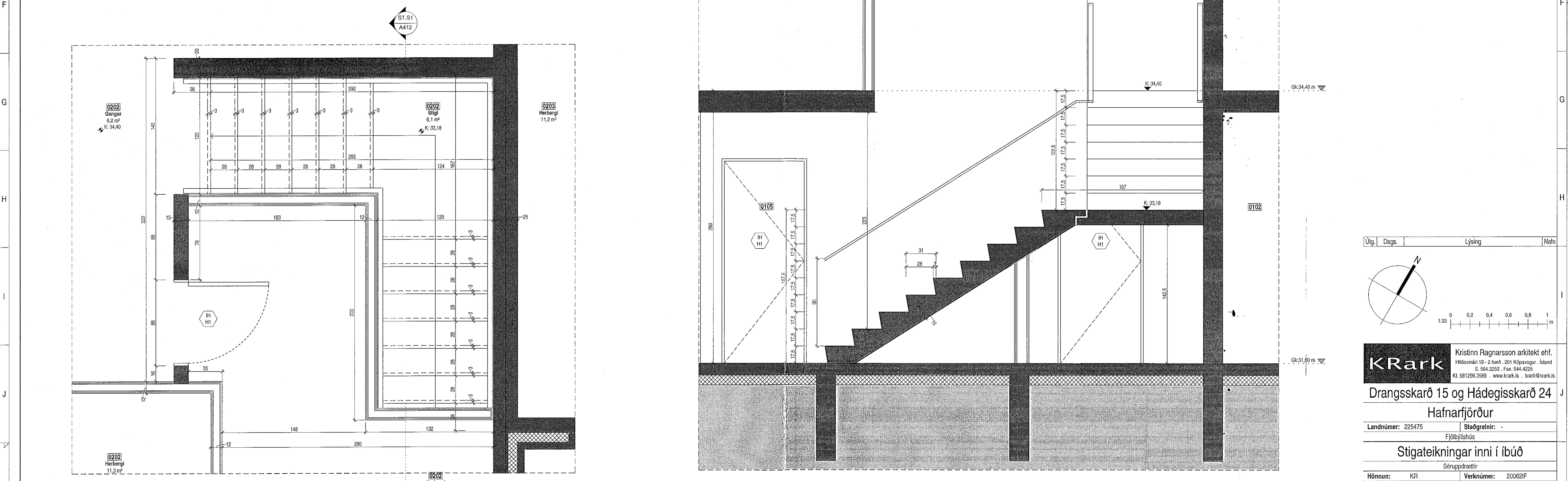
Stigateikningar Grunnmynd 2.hæð 1:20
