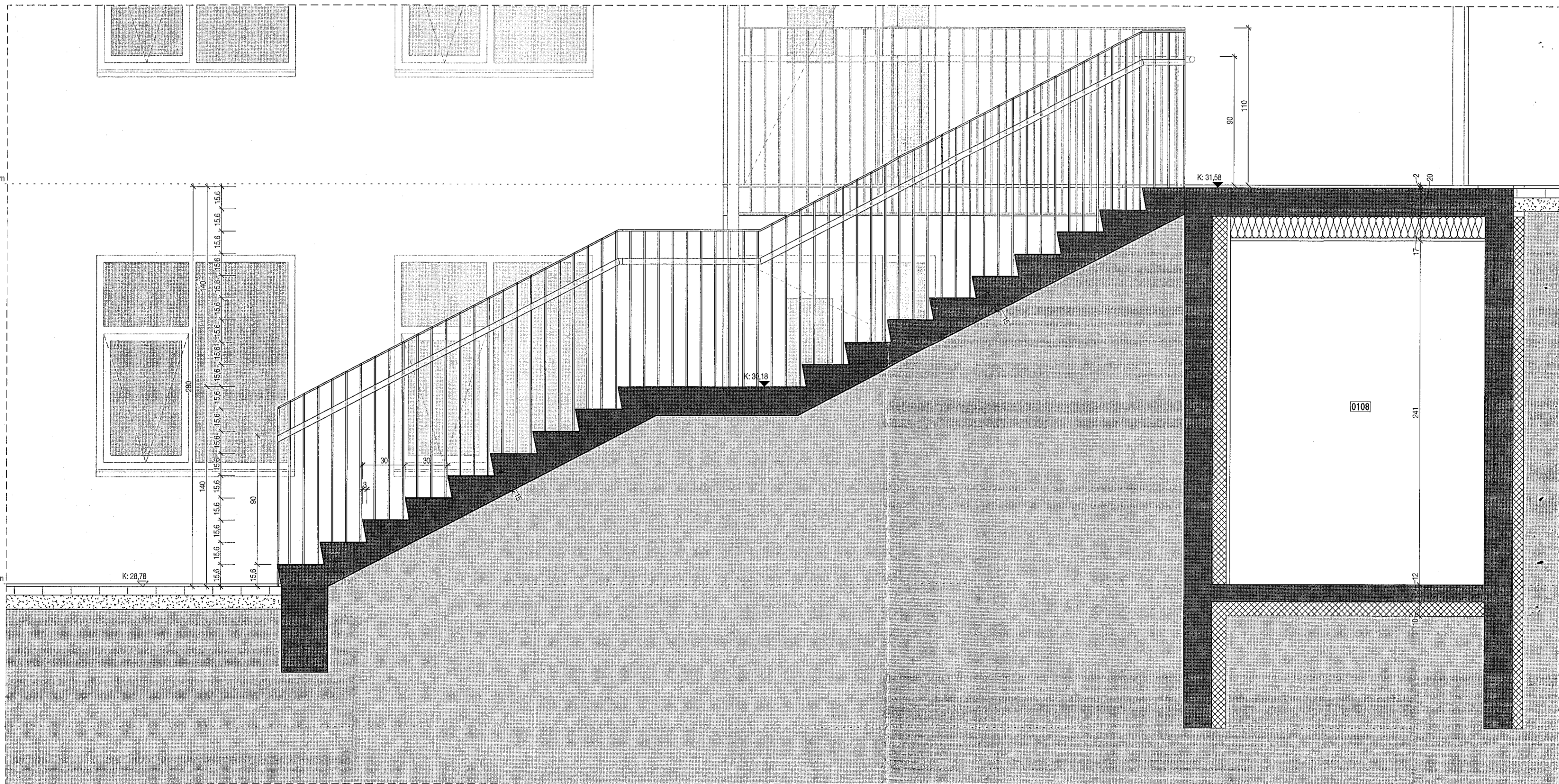
Útitróppur Snið 1:20
