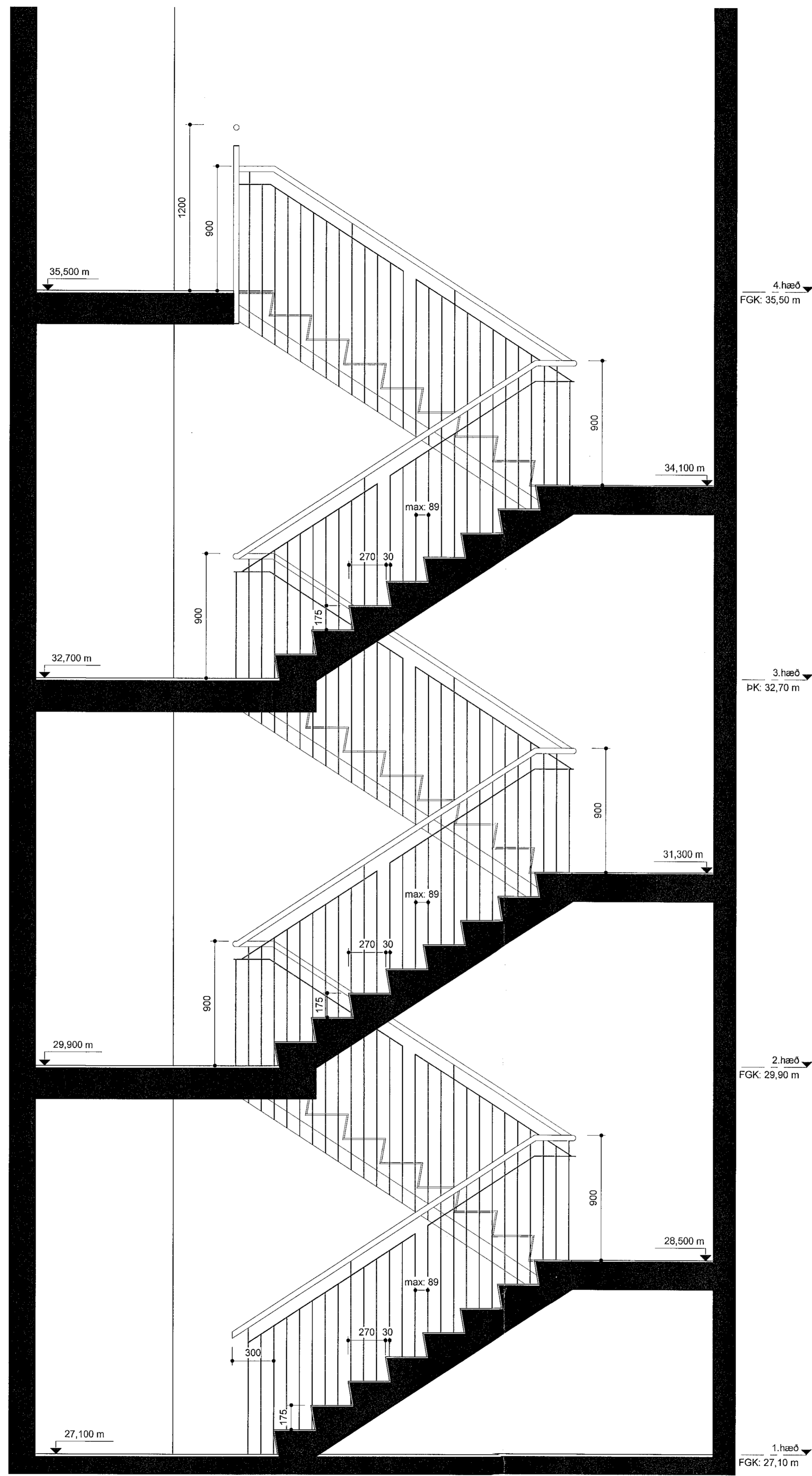
Stigi 2 - Snið 2-2
