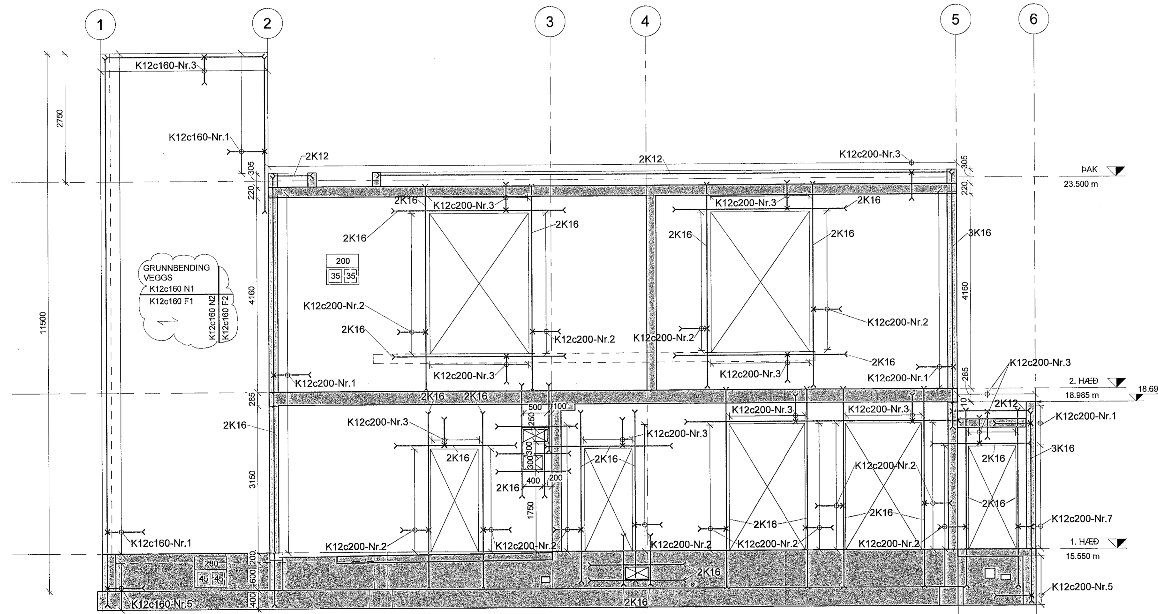
V1 ÁSÝND 101 1 : 50
