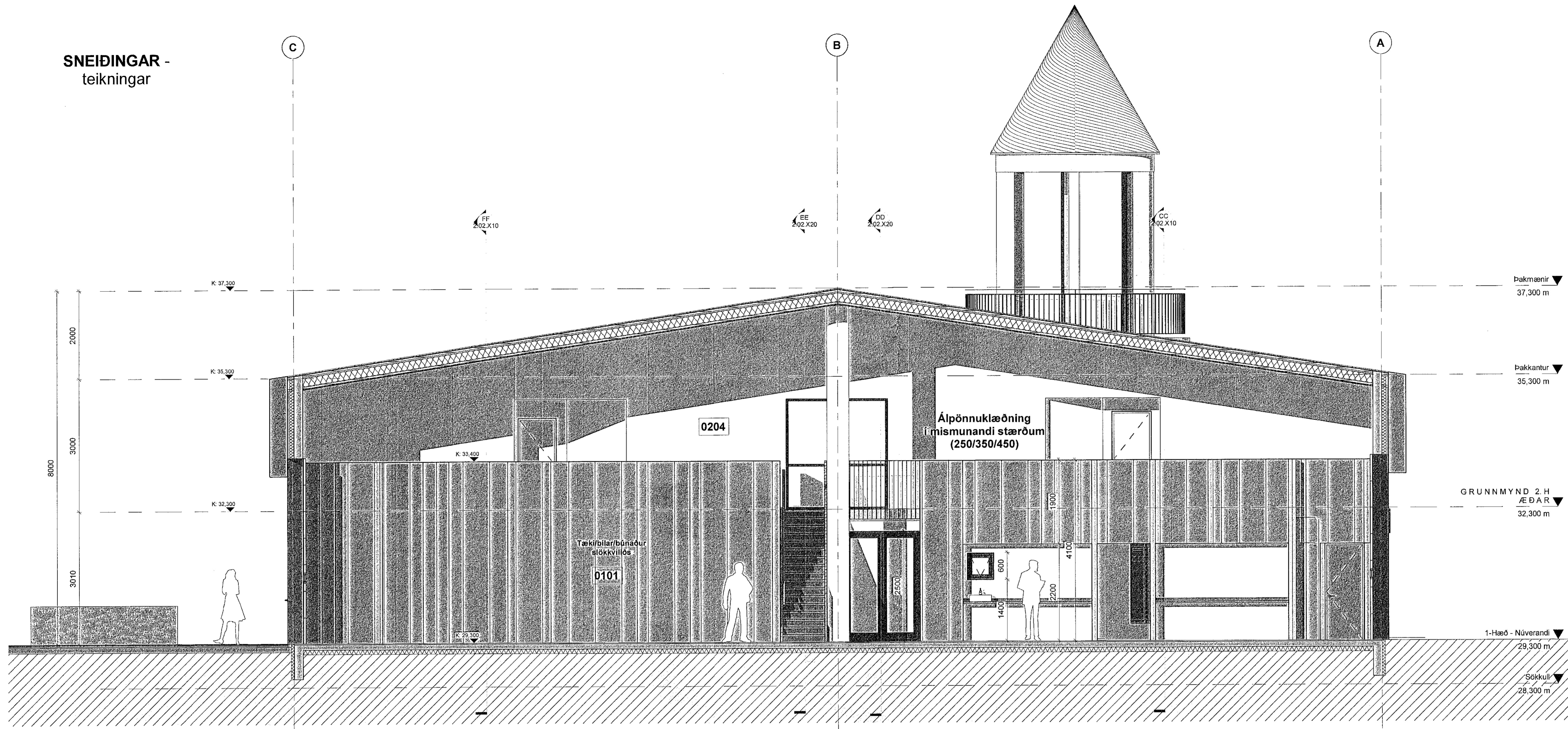
SNEIÐING AA 1:50
