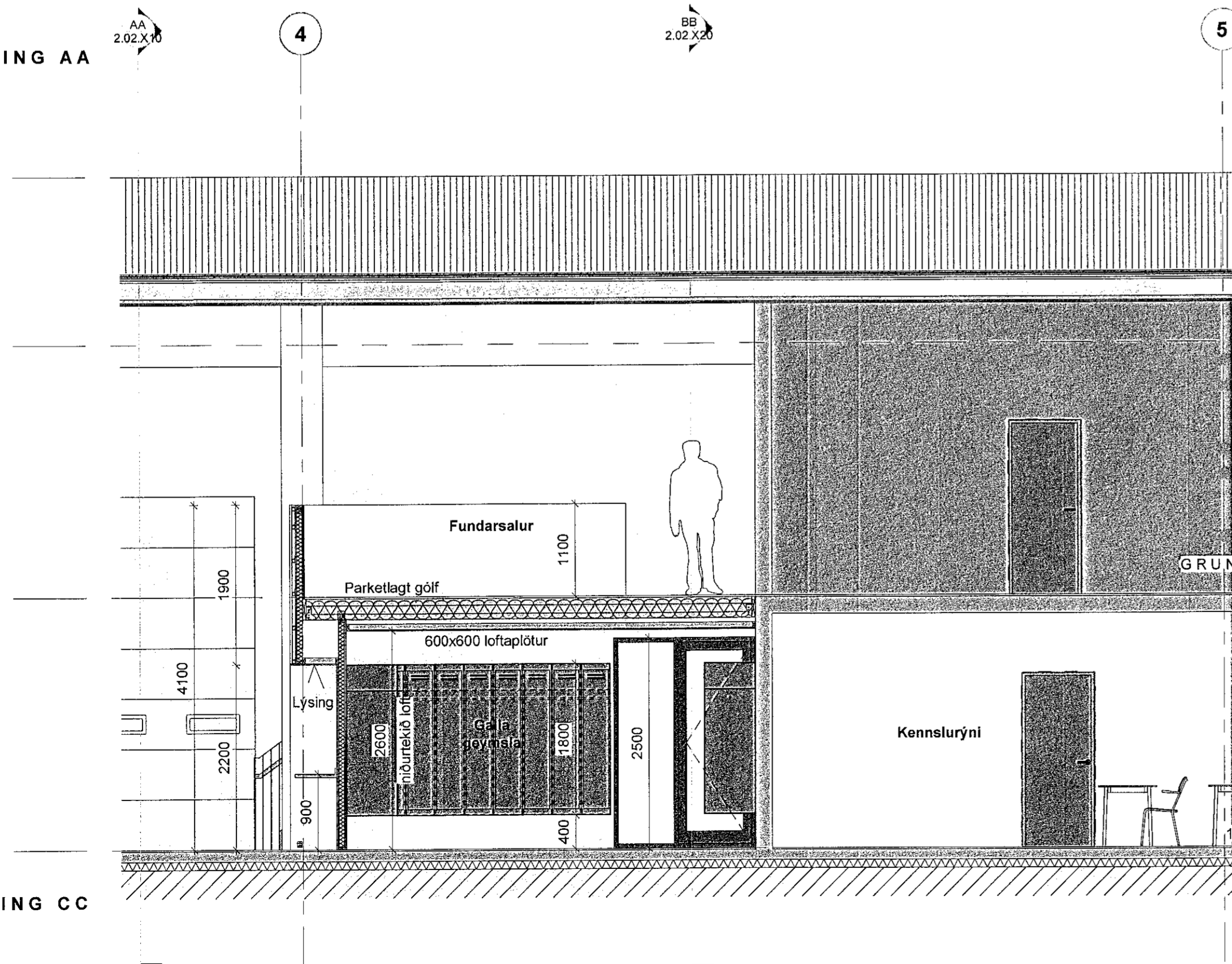
SNEIÐING FF 1:50
