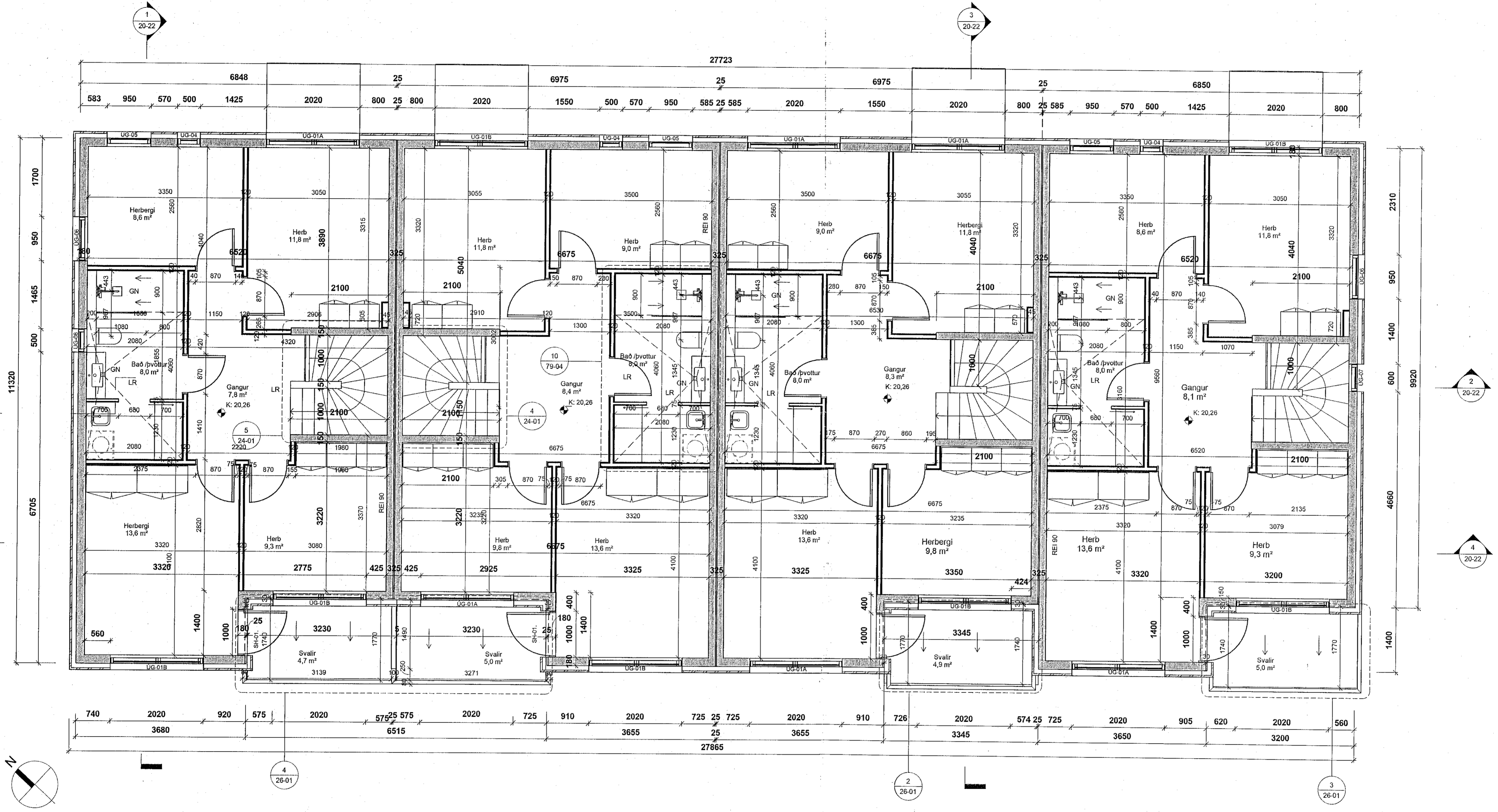
2.hæð 1.50 - (mhl 02) 1:50
