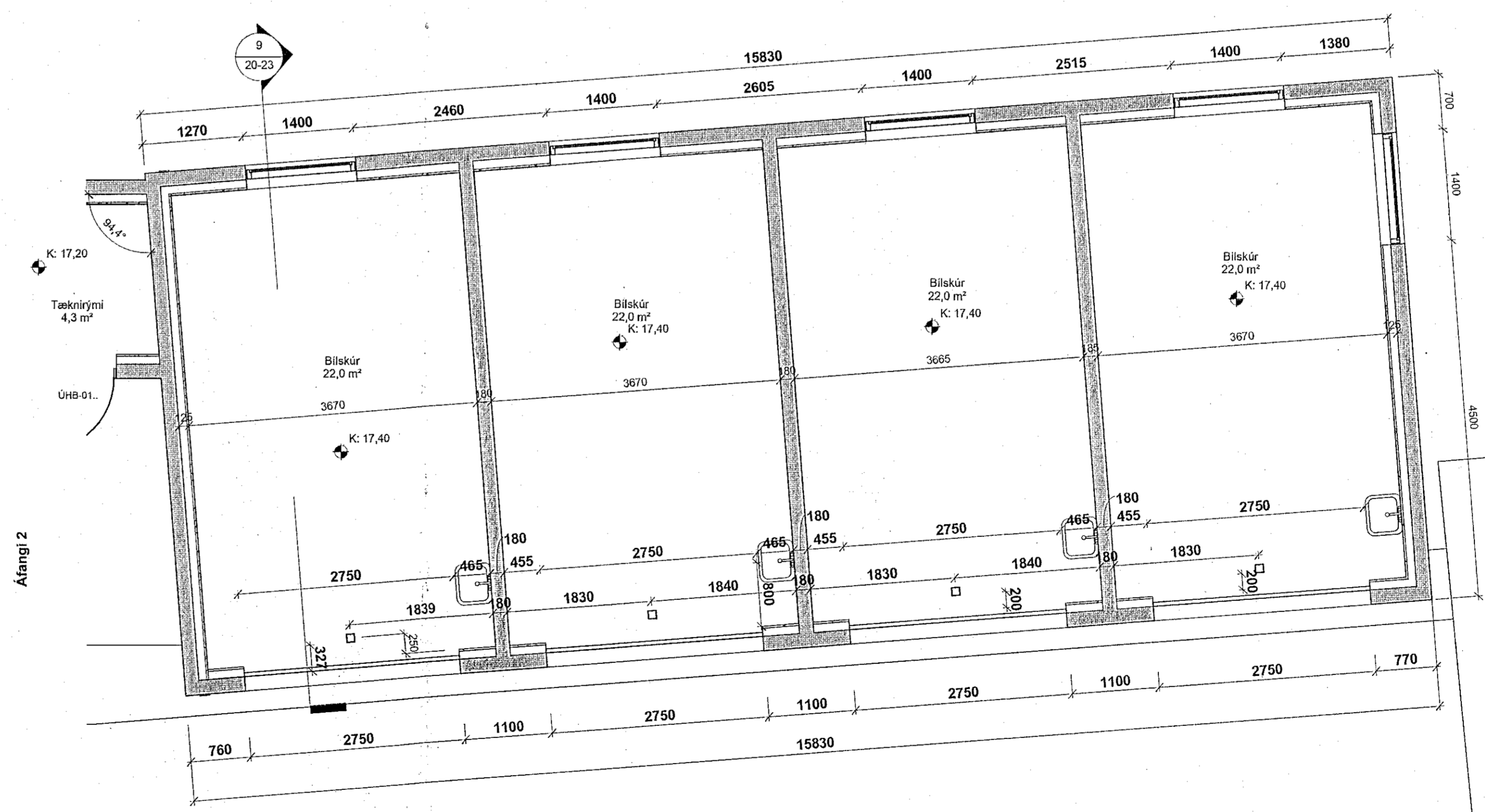
1. hæð Bílskúr (mhl 05.) 1.50 1 : 50
