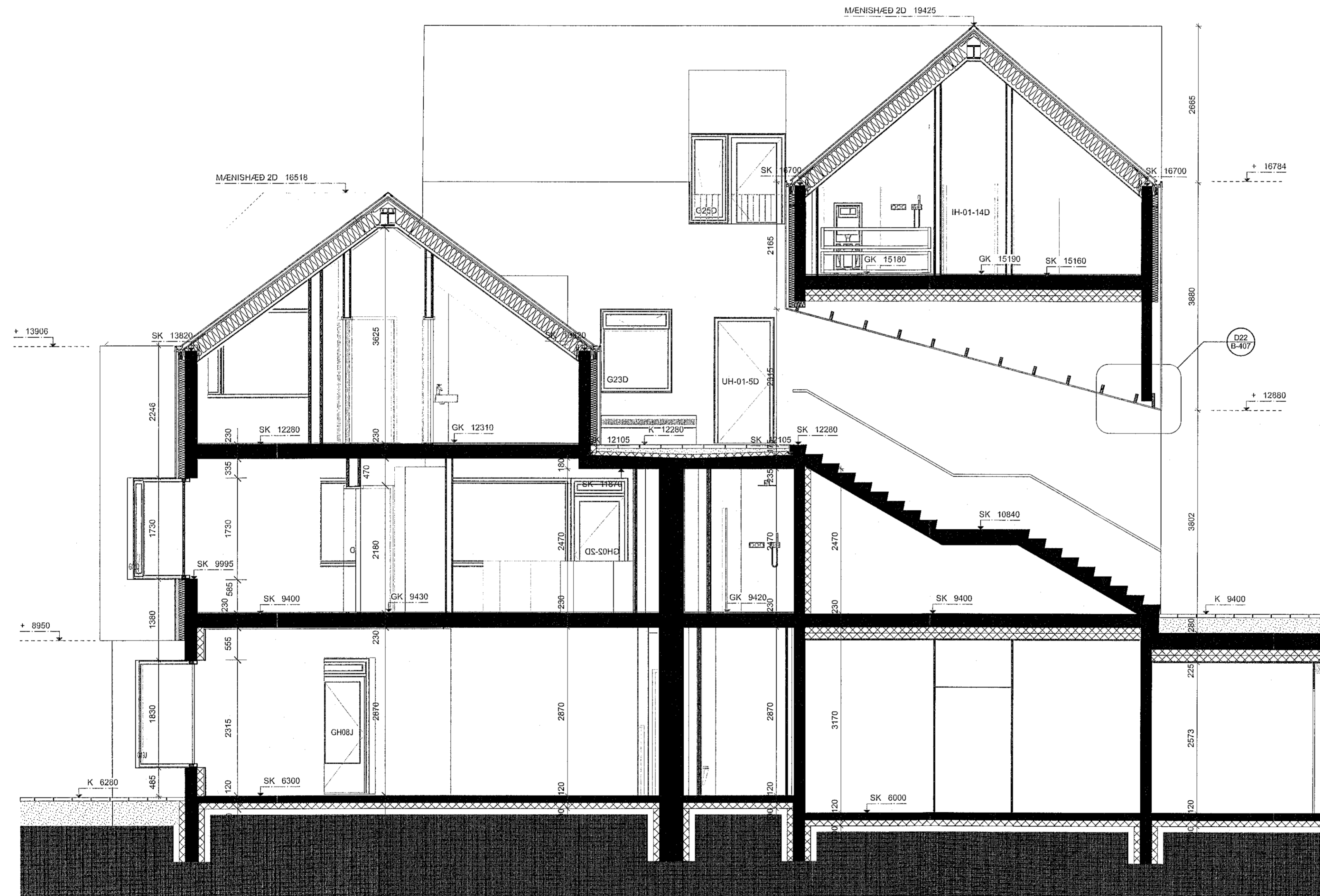
D1 Sneiðing D1 Skali: 1:50
