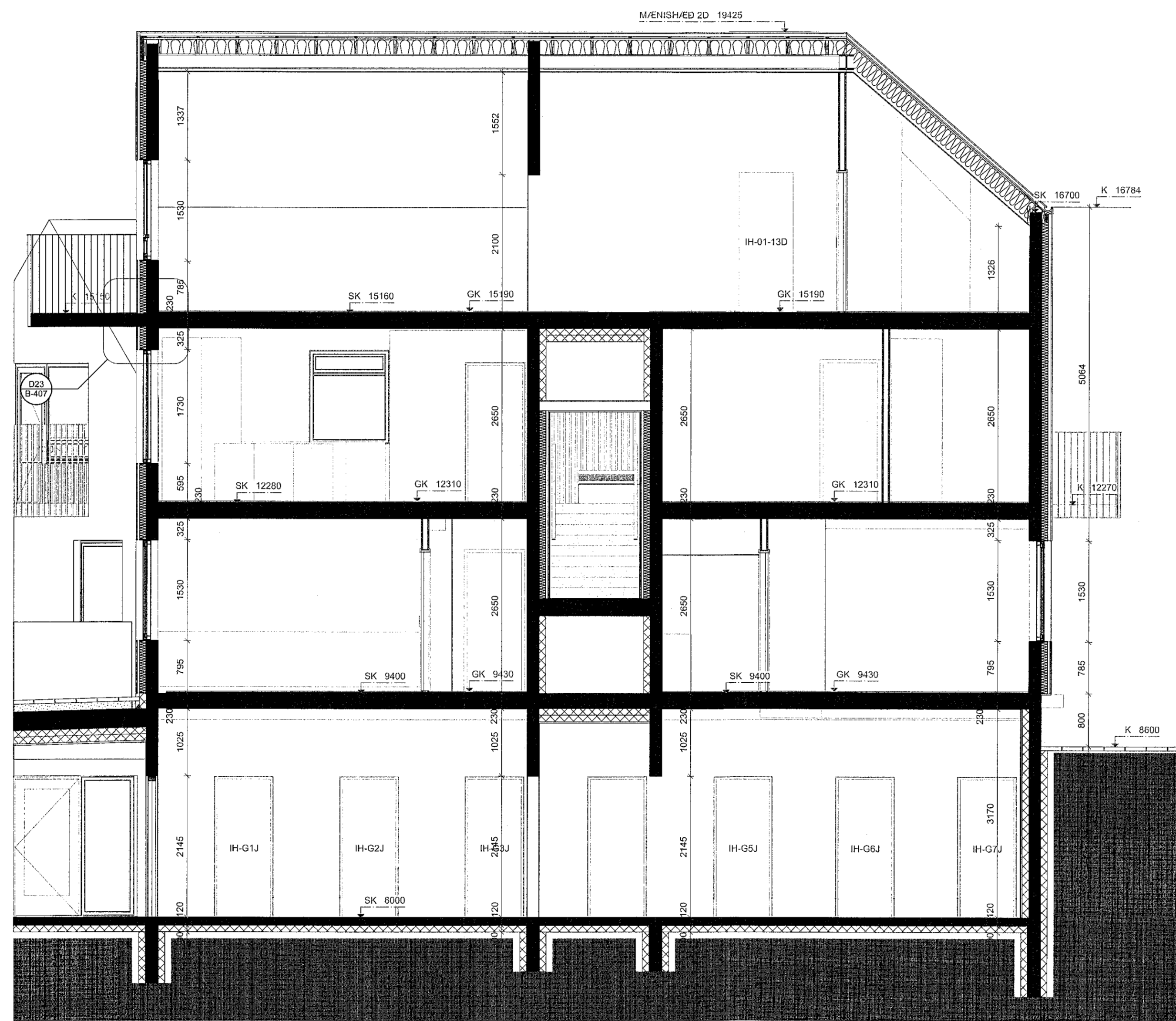
D2 SNEIDING D2 Skali: 1:50
