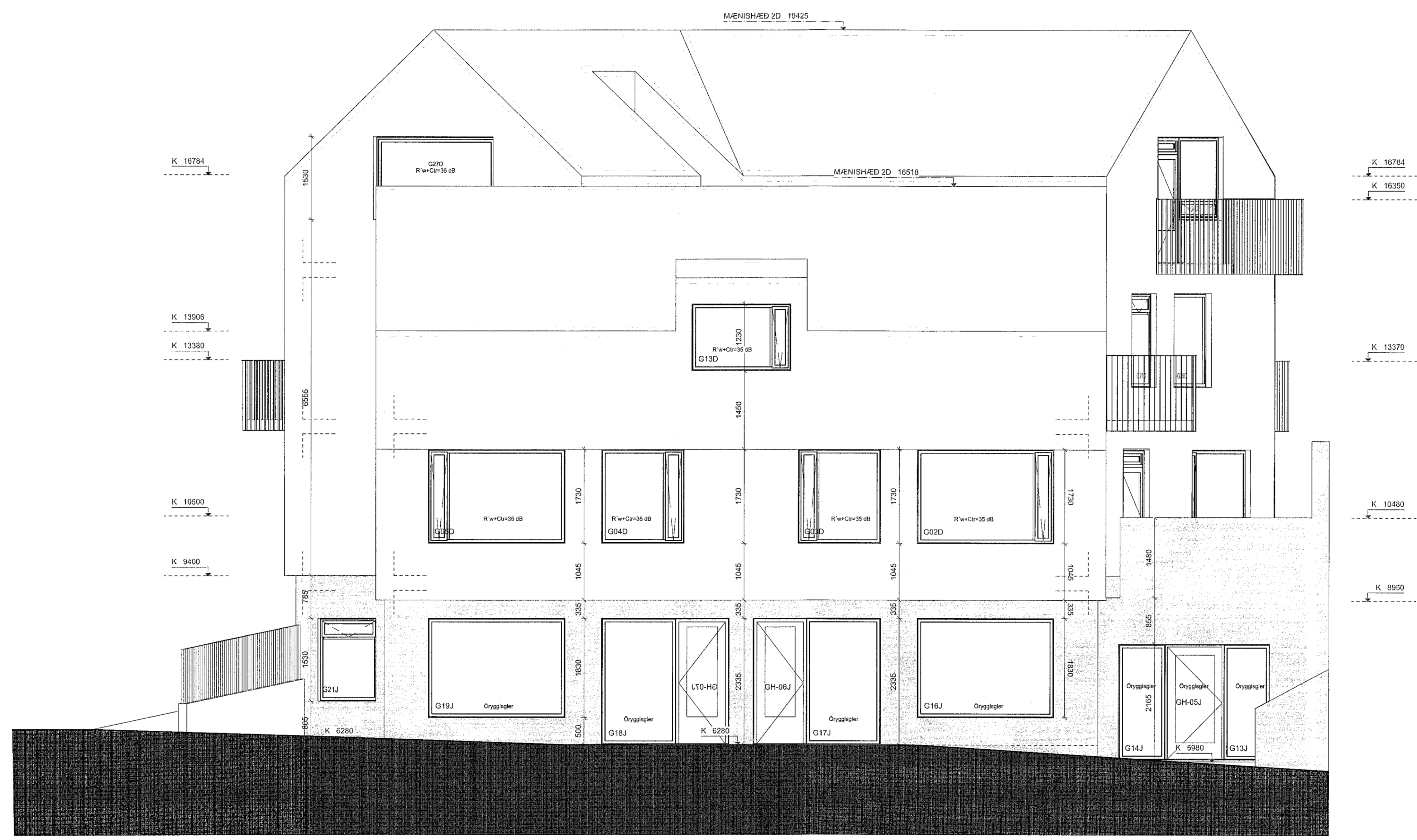
2 2D ÚTLIT NORDUR Skali: 1:50
