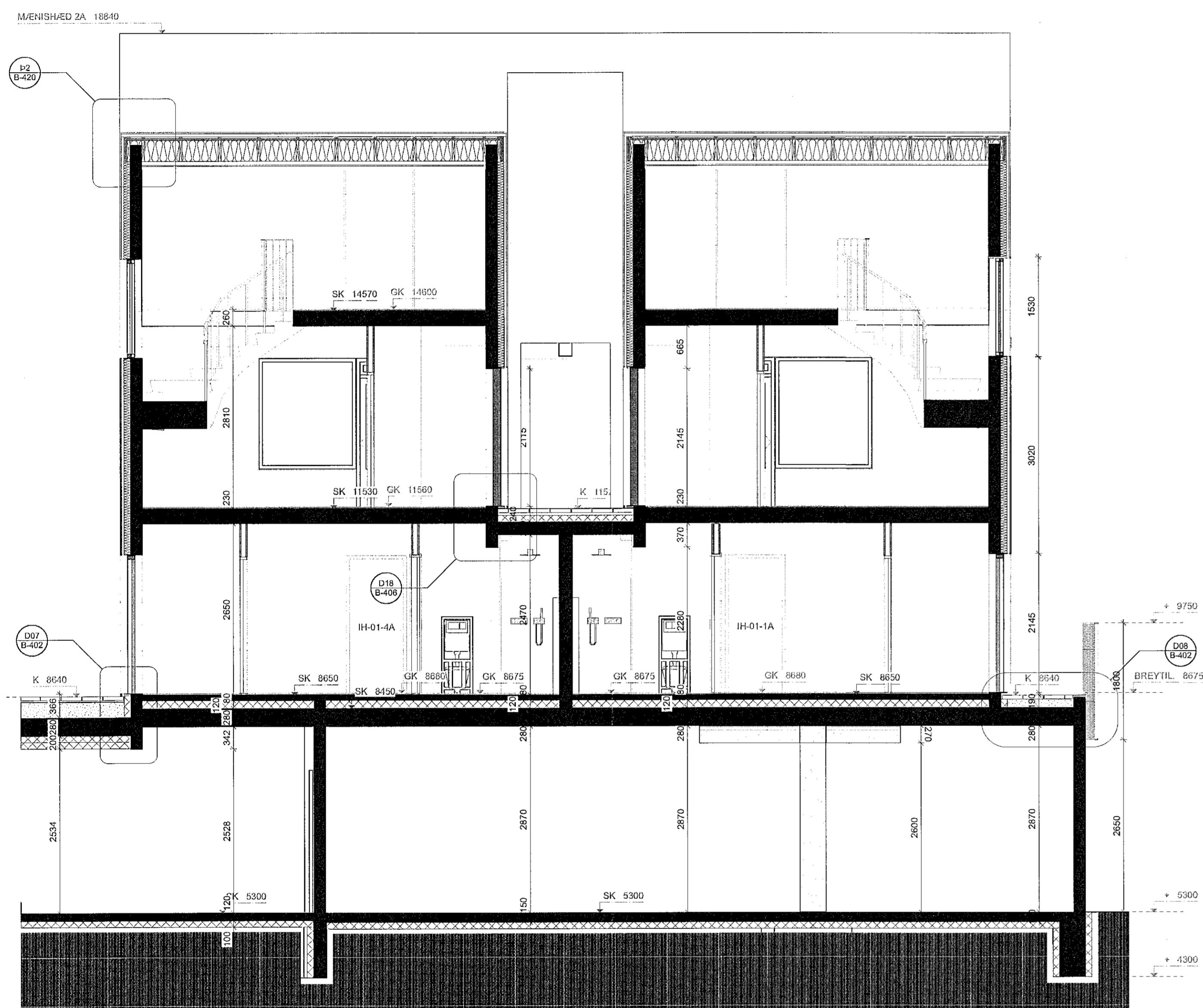
A1 SNEIÐING A1 Skali: 1:50
