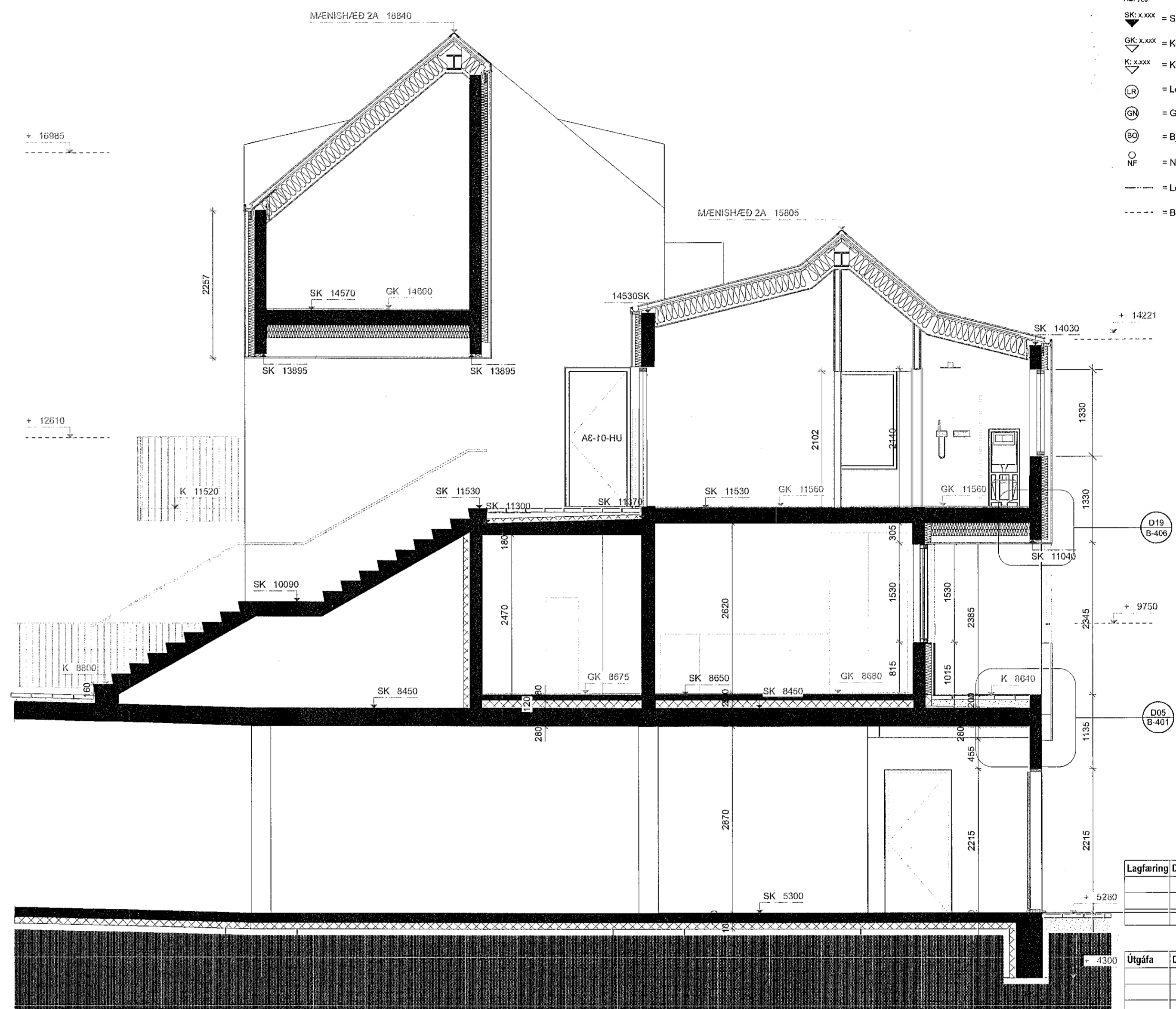
A2 SNEIÐING A2 Skali: 1:50
