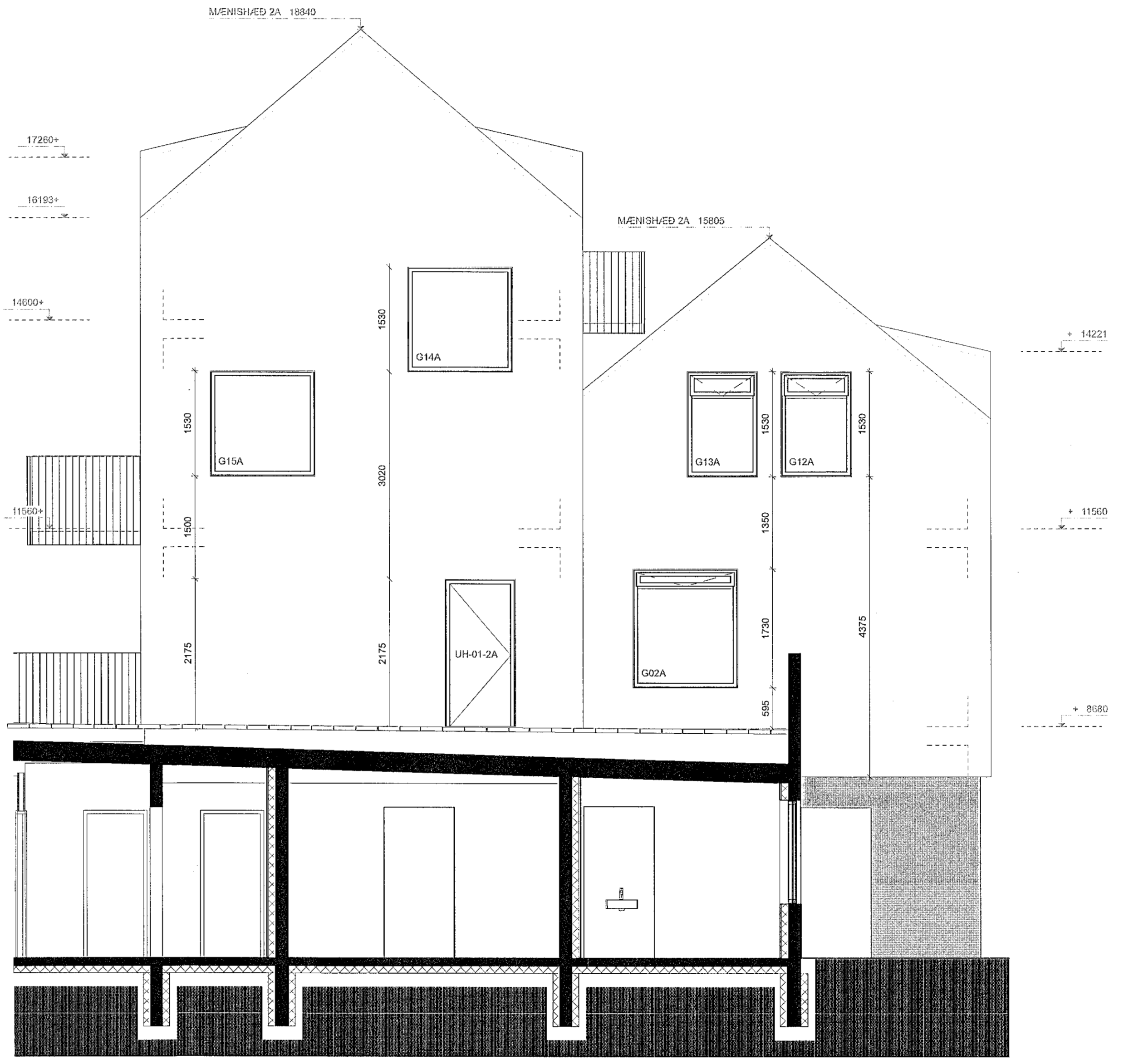
4 ÚTLIT NORDUR Skali: 1:50
