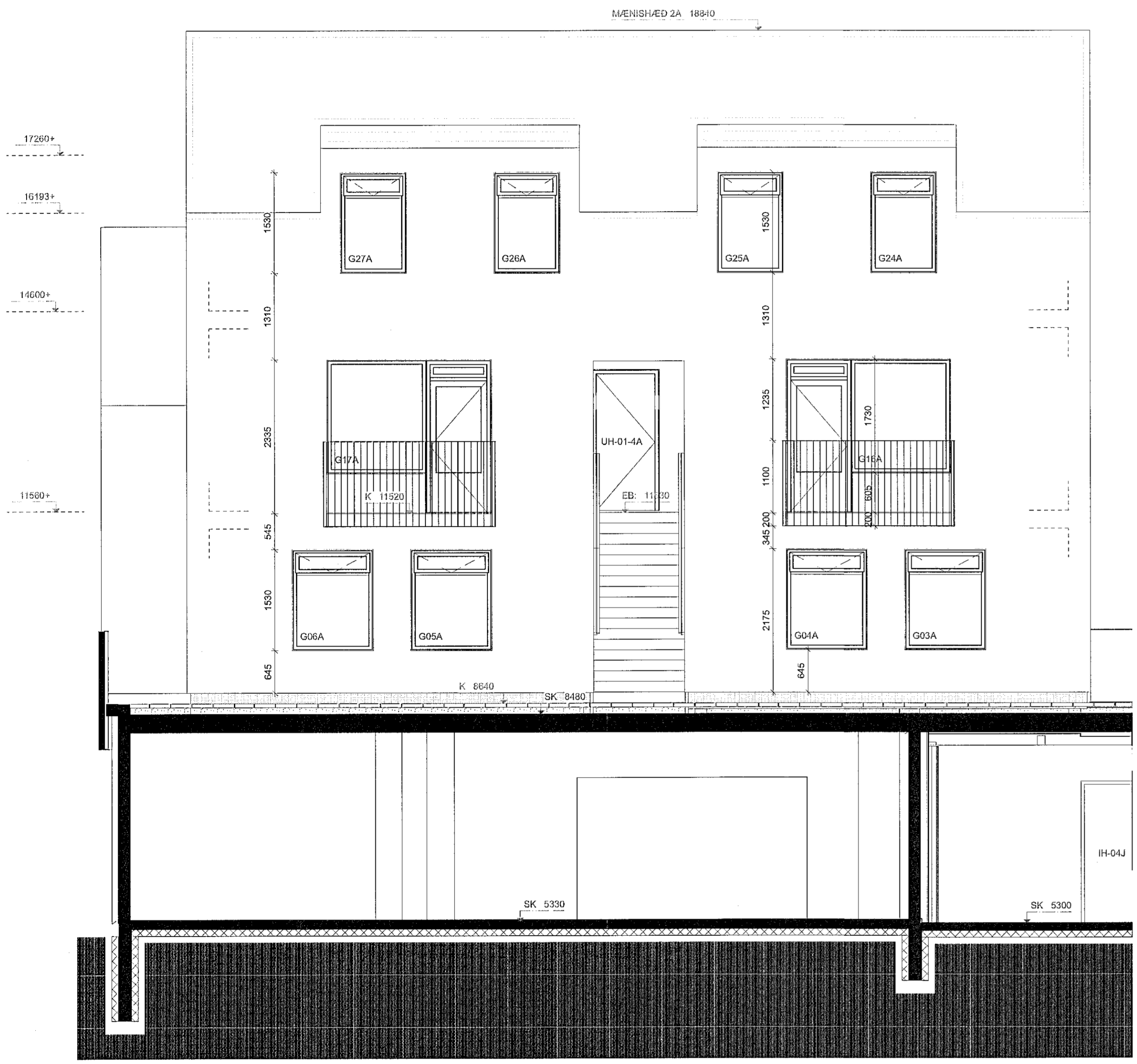
3 ÚTLIT 2AAUSTUR Skali: 1:50
