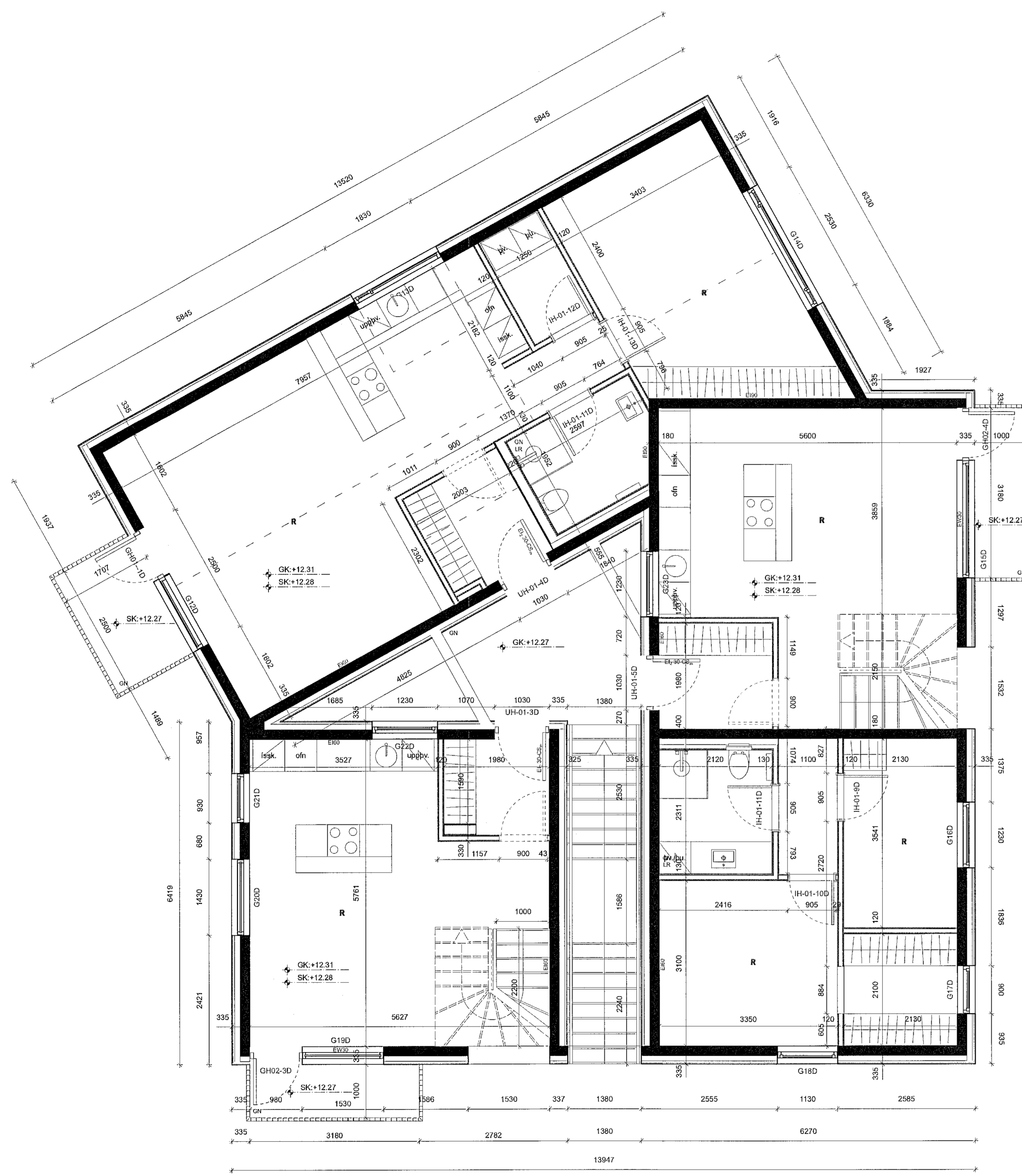
17 GRUNNMYND +3 (D-HÚS) Skali: 1:50
