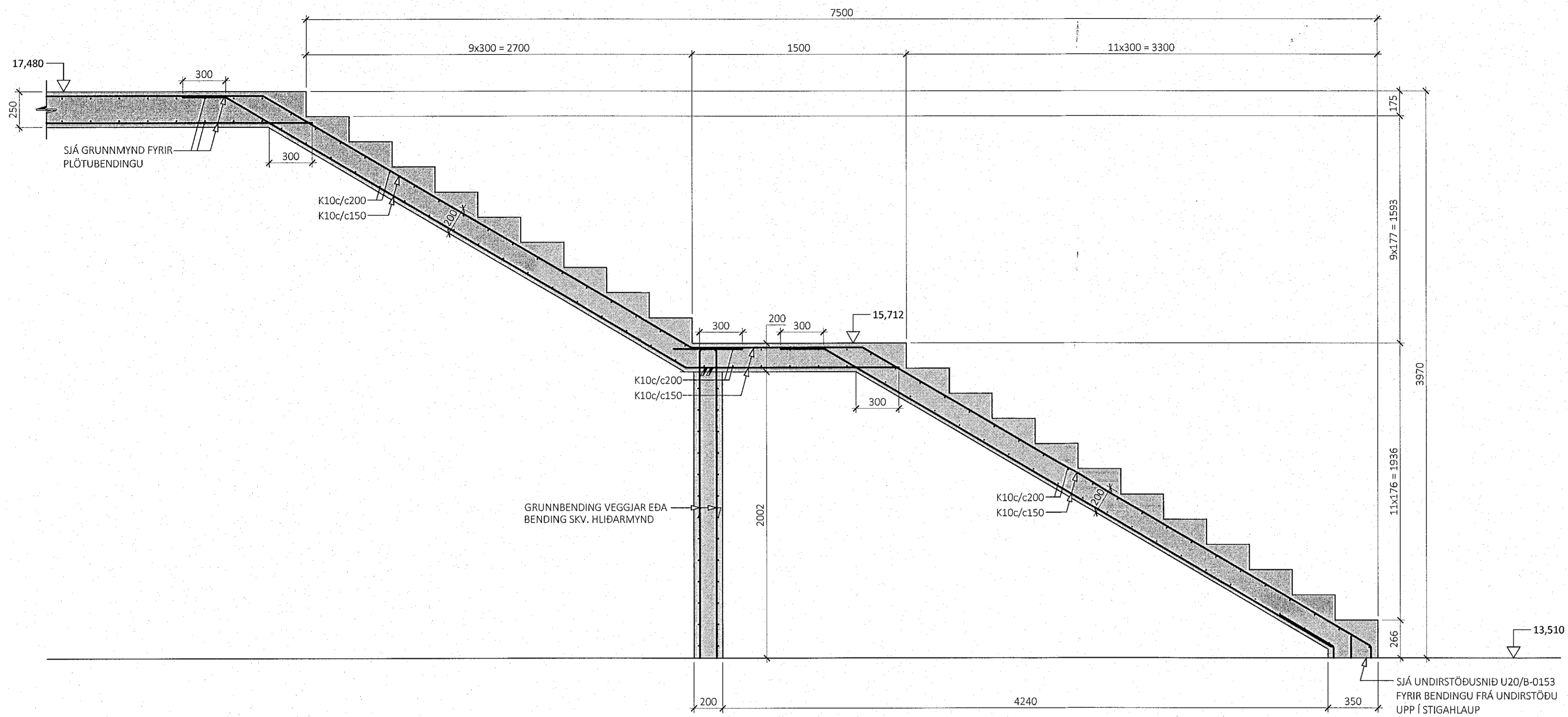
ALMENNT SNIÐ FYRIR ENDAFRÁGANG Á TRÖPPUM
