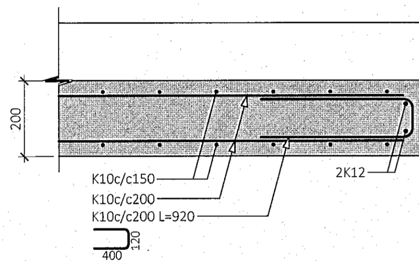
ALMENNT SNIÐ FYRIR ENDAFRÁGANG Á TRÖPPUM
